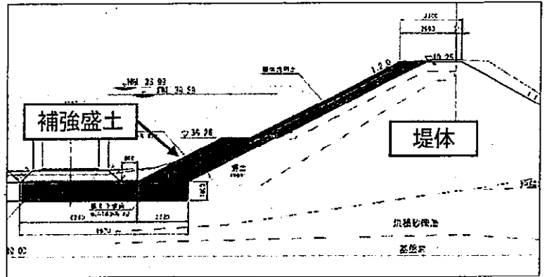
耐震補強計画断面図
