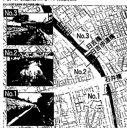
河川内通路工事の概要図
