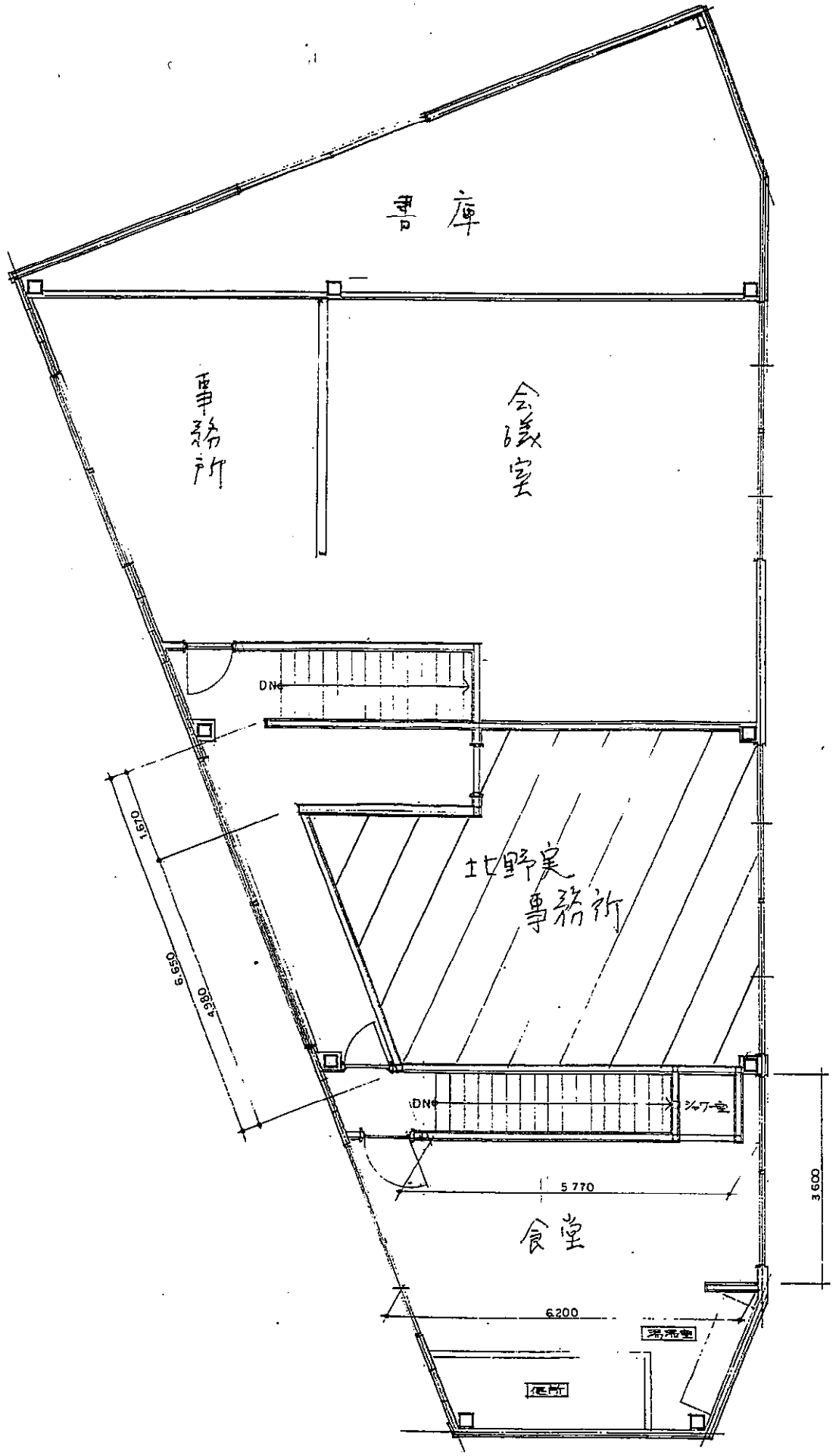
2階平面図
