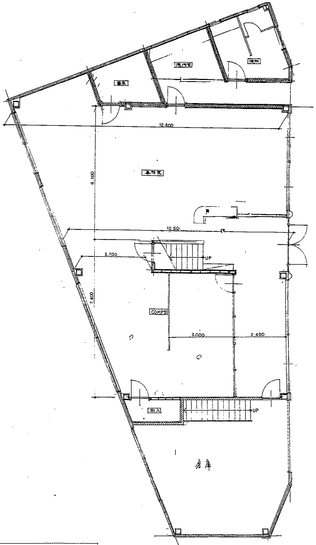
1階平面図
