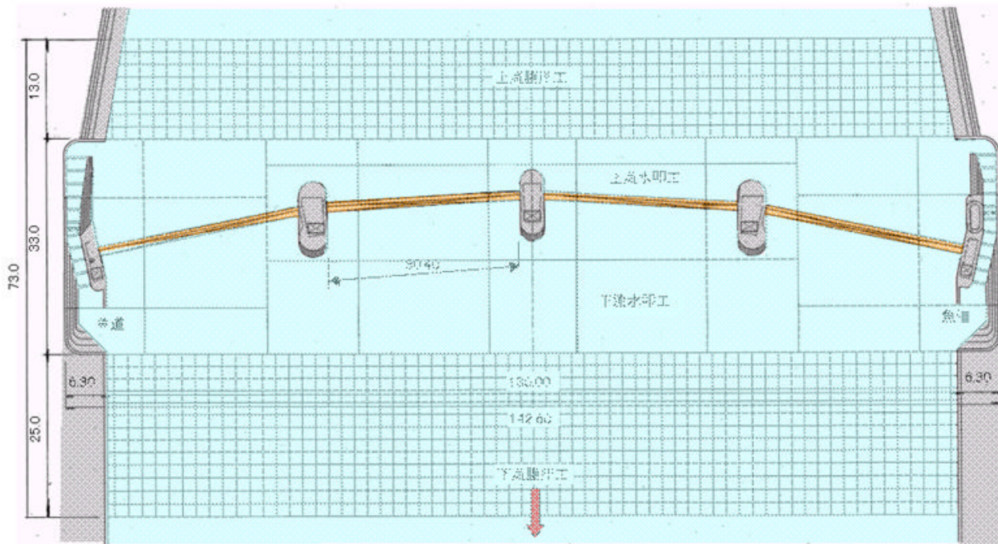
一般平面図
