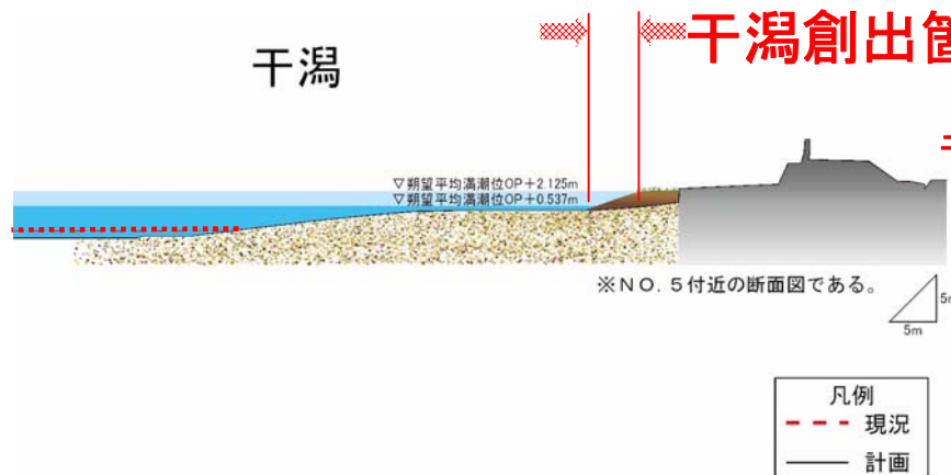
横断面図
