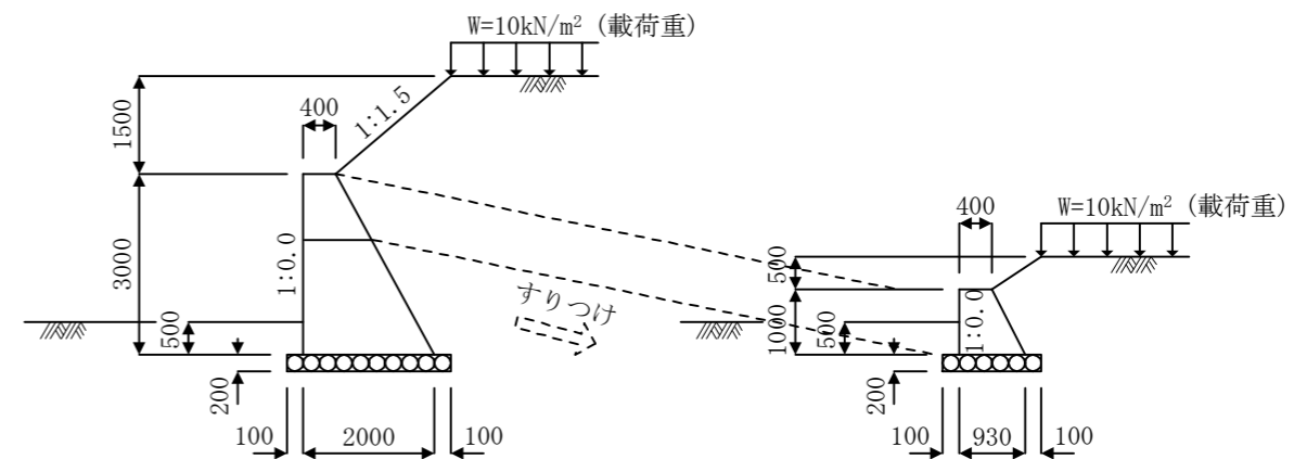
図-15 断面図
