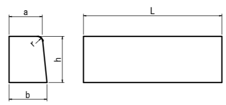
歩車道境界ブロック(JIS)
