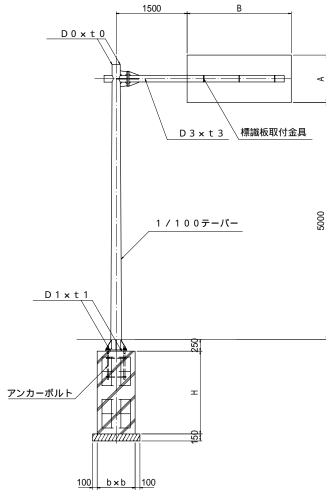
寸法表
