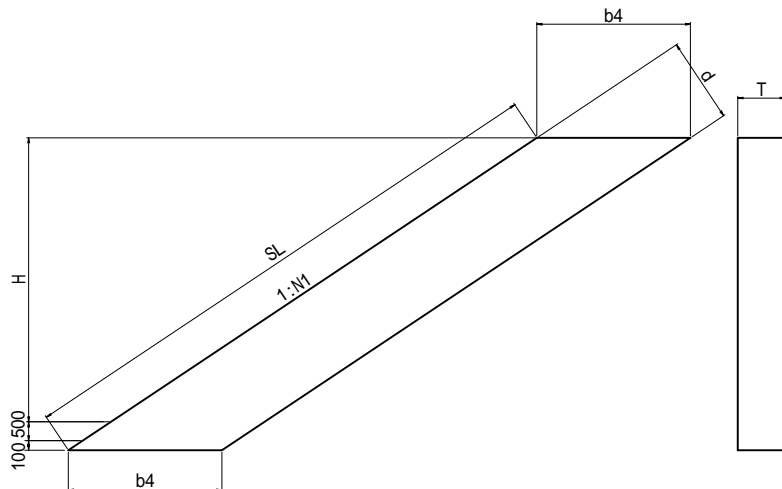
コンクリートブロック張用 (平板ブロック a = 1 8 0 mm、練張りブロック a = 3 5 0 mm)
