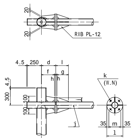
柱，梁接合部詳細図
