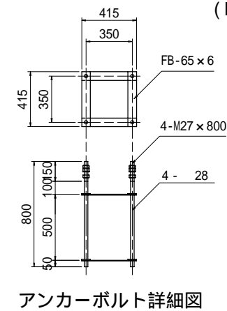
ベースプレート詳細図
