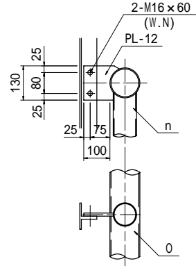
標識板取付金具詳細図
