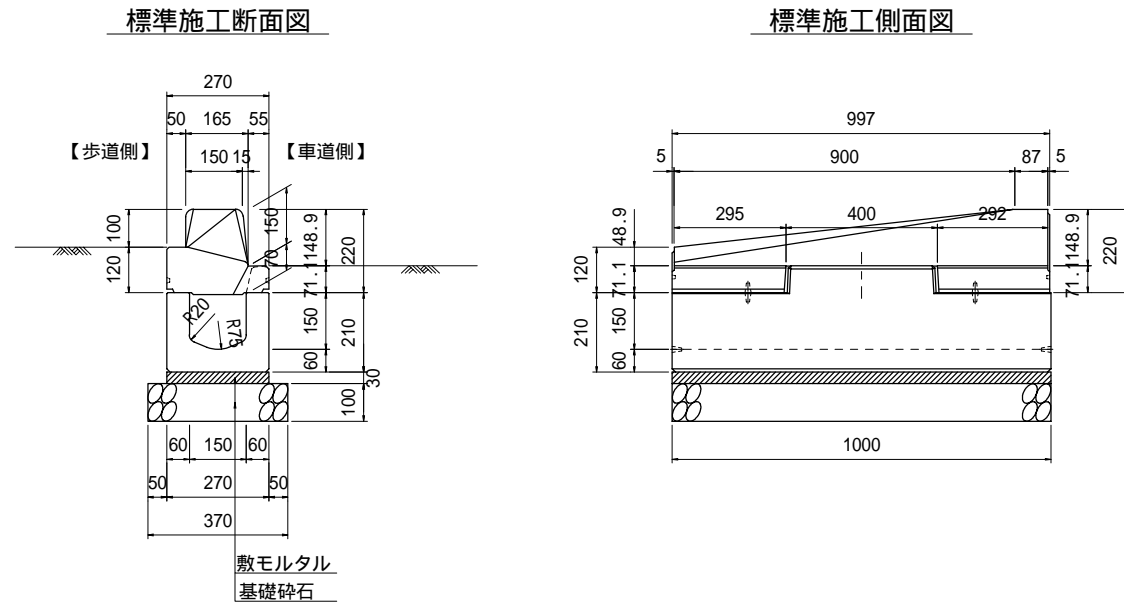
擦付部 (150×150) (標準部 A 型 - 車両乗入部)
