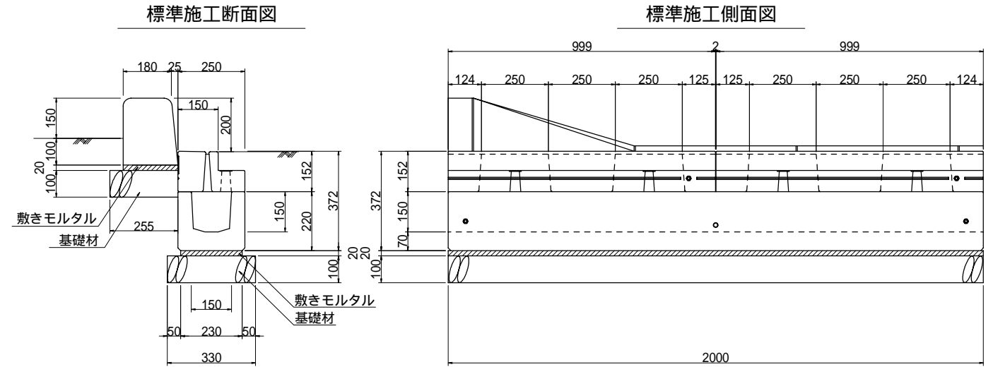
擦付部 (150型) (標準部B型 - 歩道切下部)
