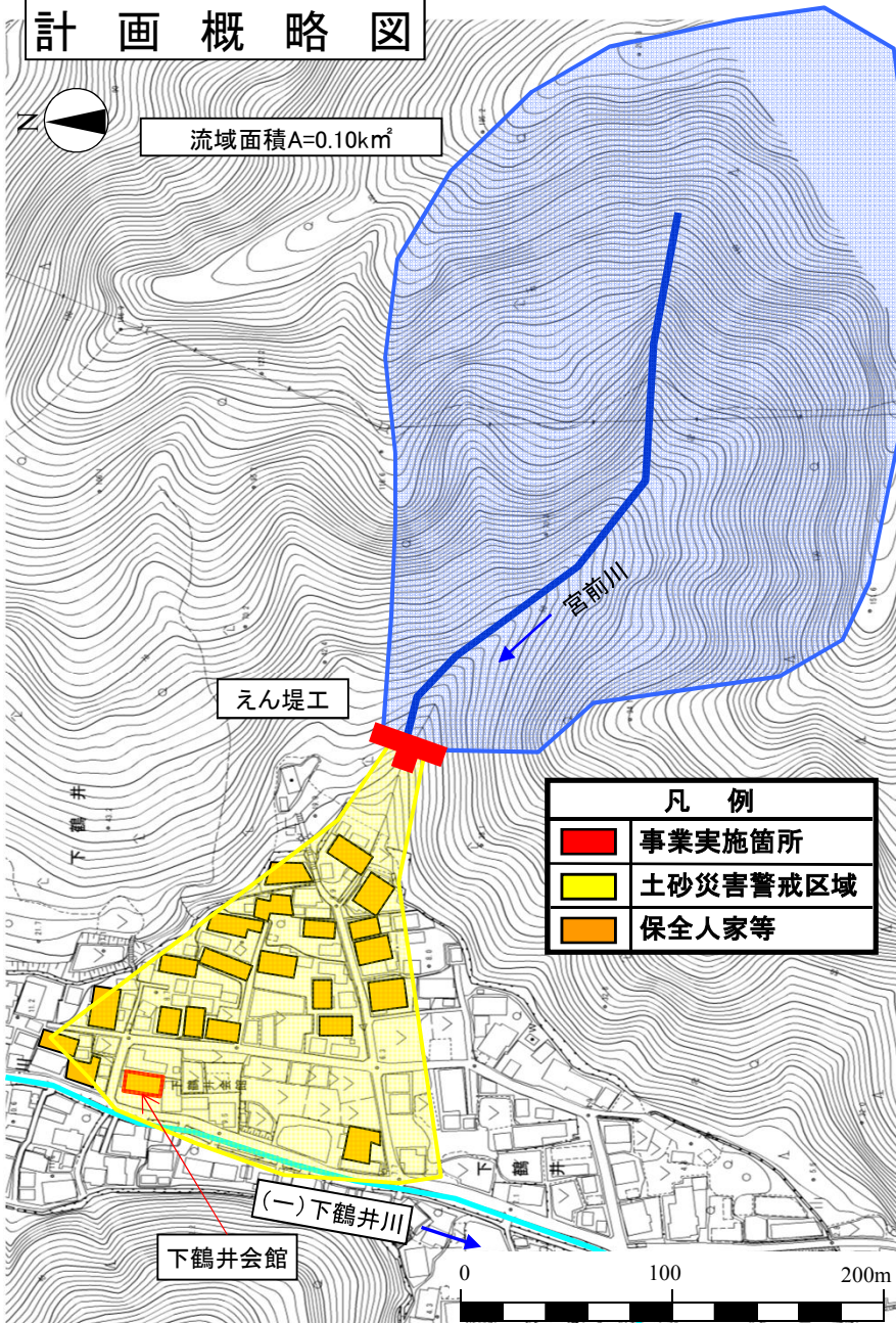
えん堤工 H=9.0m、L=40.0m
