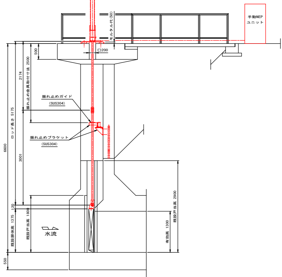
断面図
