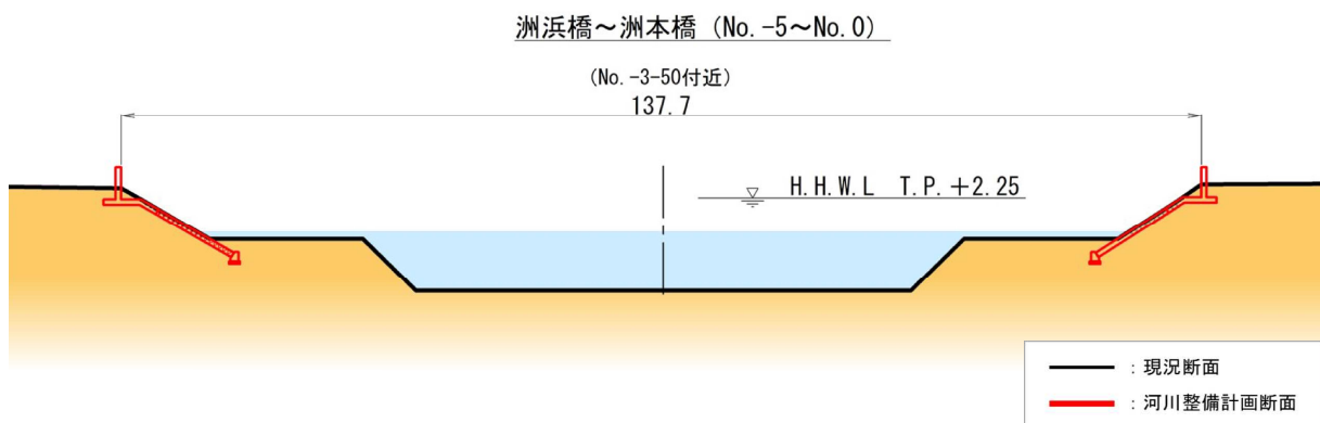
図 2.1.5 高潮対策の標準断面
