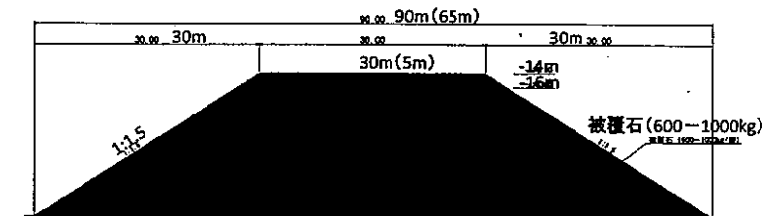
海底地盤 -34m NO.1長辺断面 ( )は短辺断面の寸法
