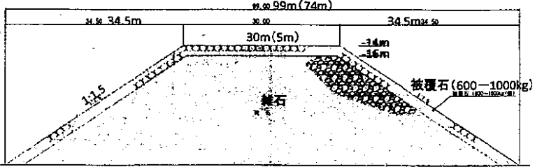
海底地盤 -37m NO.3長辺断面 ( )は短辺断面の寸法
