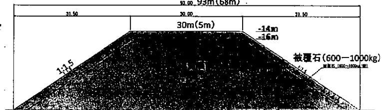
海底地盤 -35m NO.2長辺断面 ( )は短辺断面の寸法
