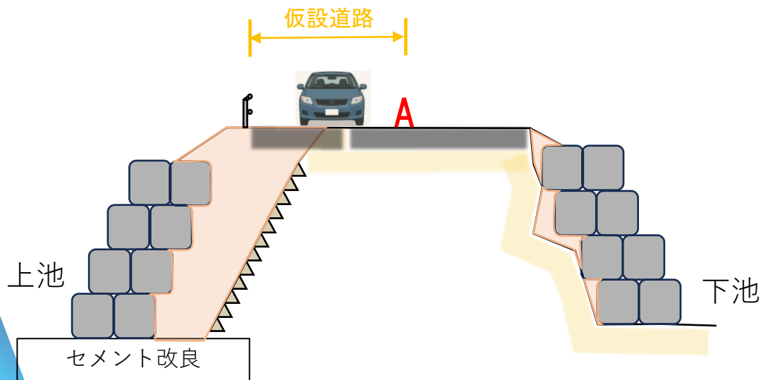
仮設道路 横断イメージ図
