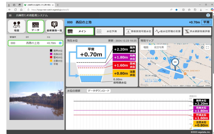
ICTを活用したため池水位の遠隔監視 (明石市)
