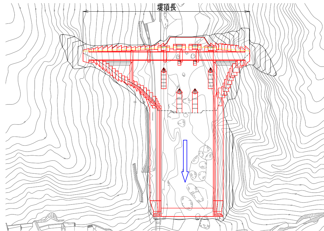
新規ダム平面図
