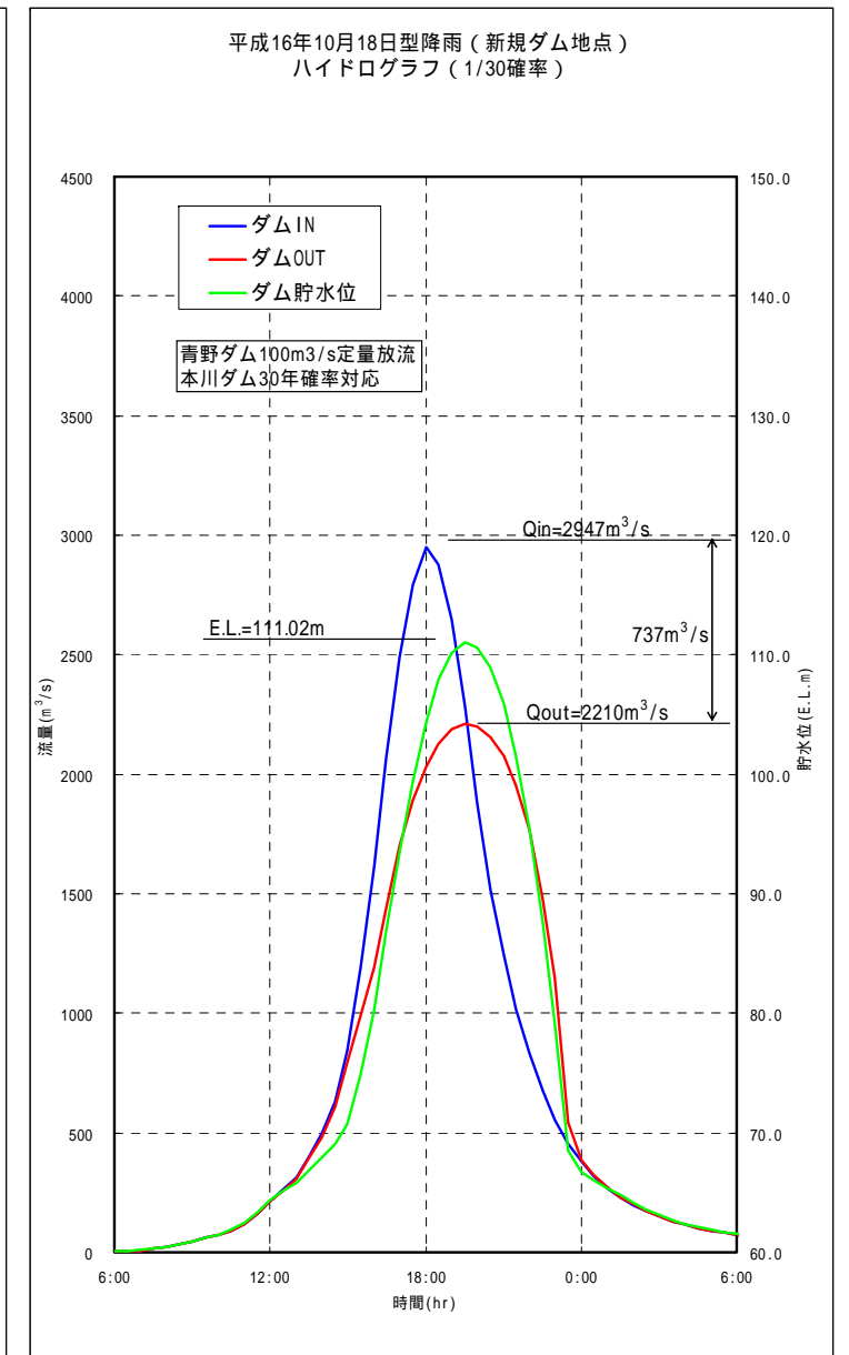
新規ダムを最適化した場合のダム地点ハイドログラフ（1/20 対応、1/30 対応）
