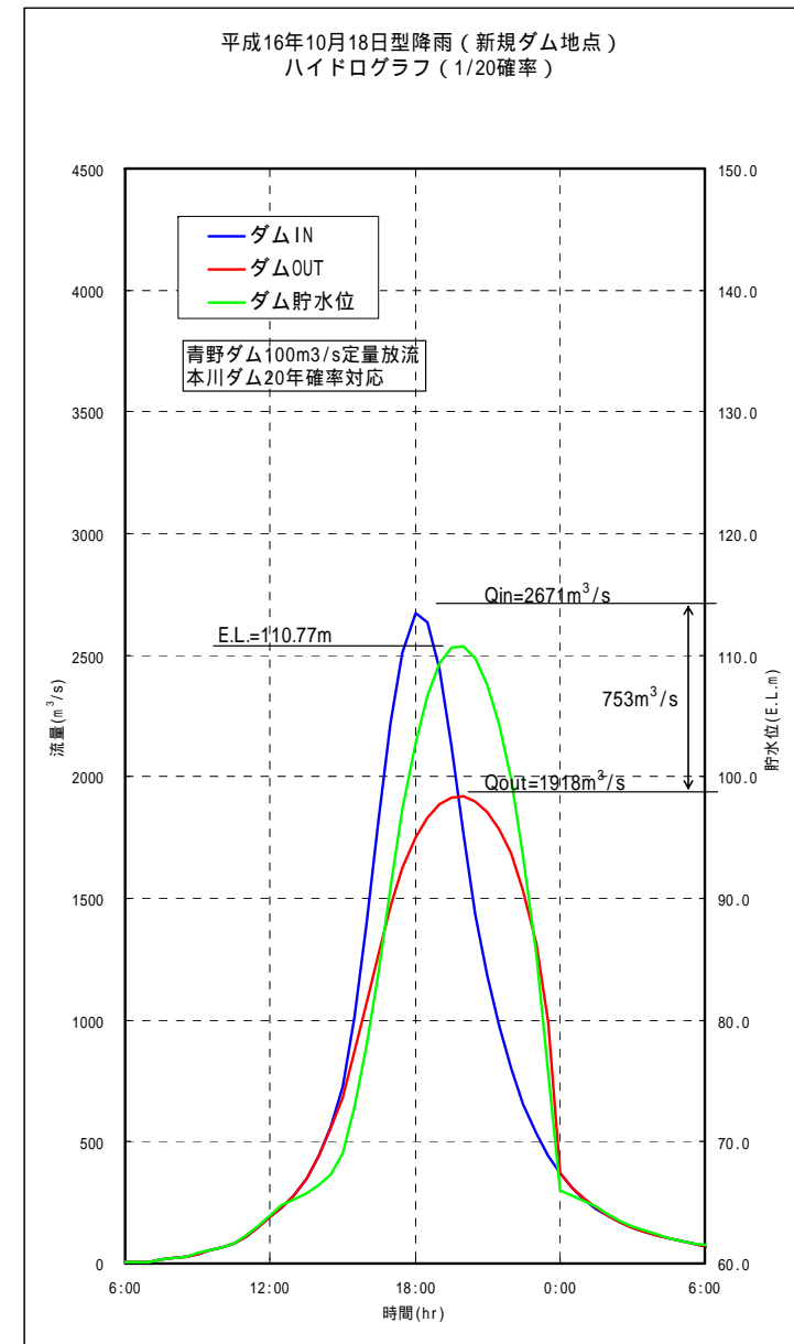
新規ダムを最適化した場合のダム地点ハイドログラフ（1/20 対応、1/30 対応）
