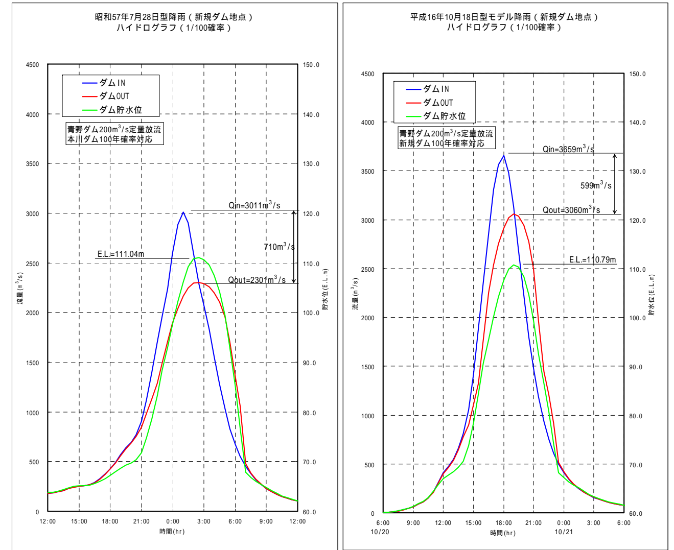
新規ダムを最適化した場合のダム地点ハイドログラフ (S57 対応、H16 対応)
