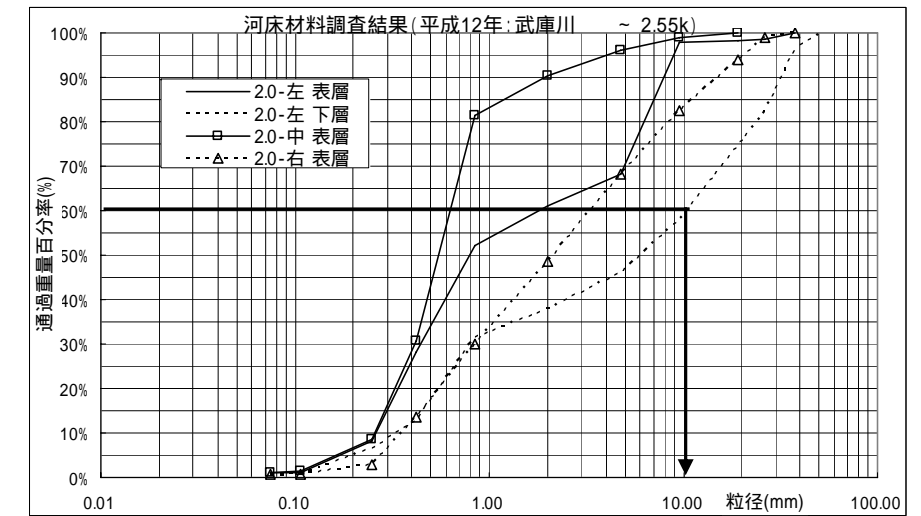
図 2.0kの河床材料調査結果
