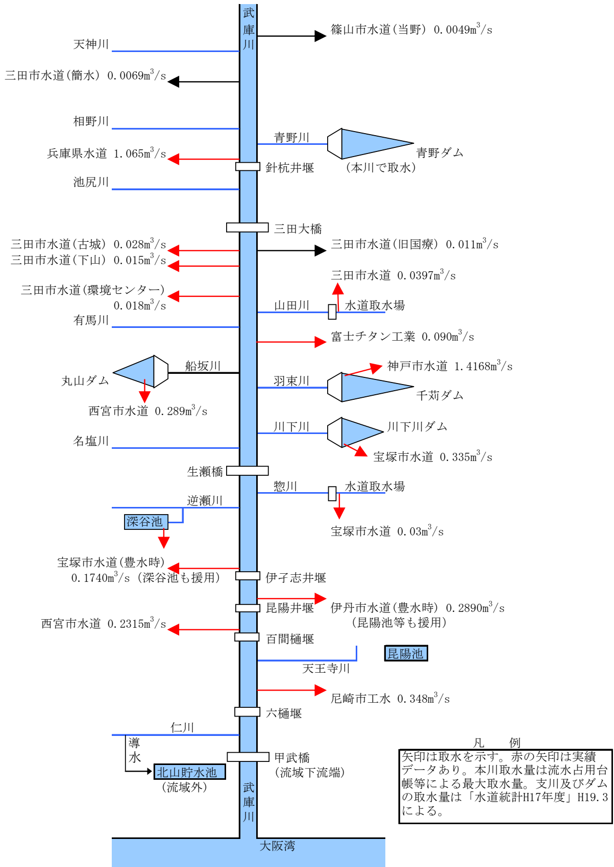
図 1.1 武庫川からの取水模式図 (主水道用水・工業用水)
