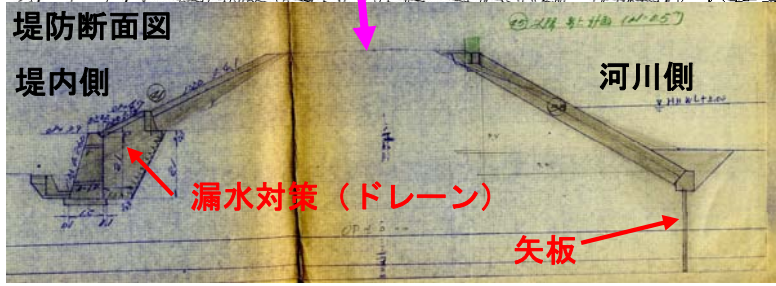
堤防強化工事の詳細調査の際、過去に施行した矢板及び漏水対策工が確認された箇所
