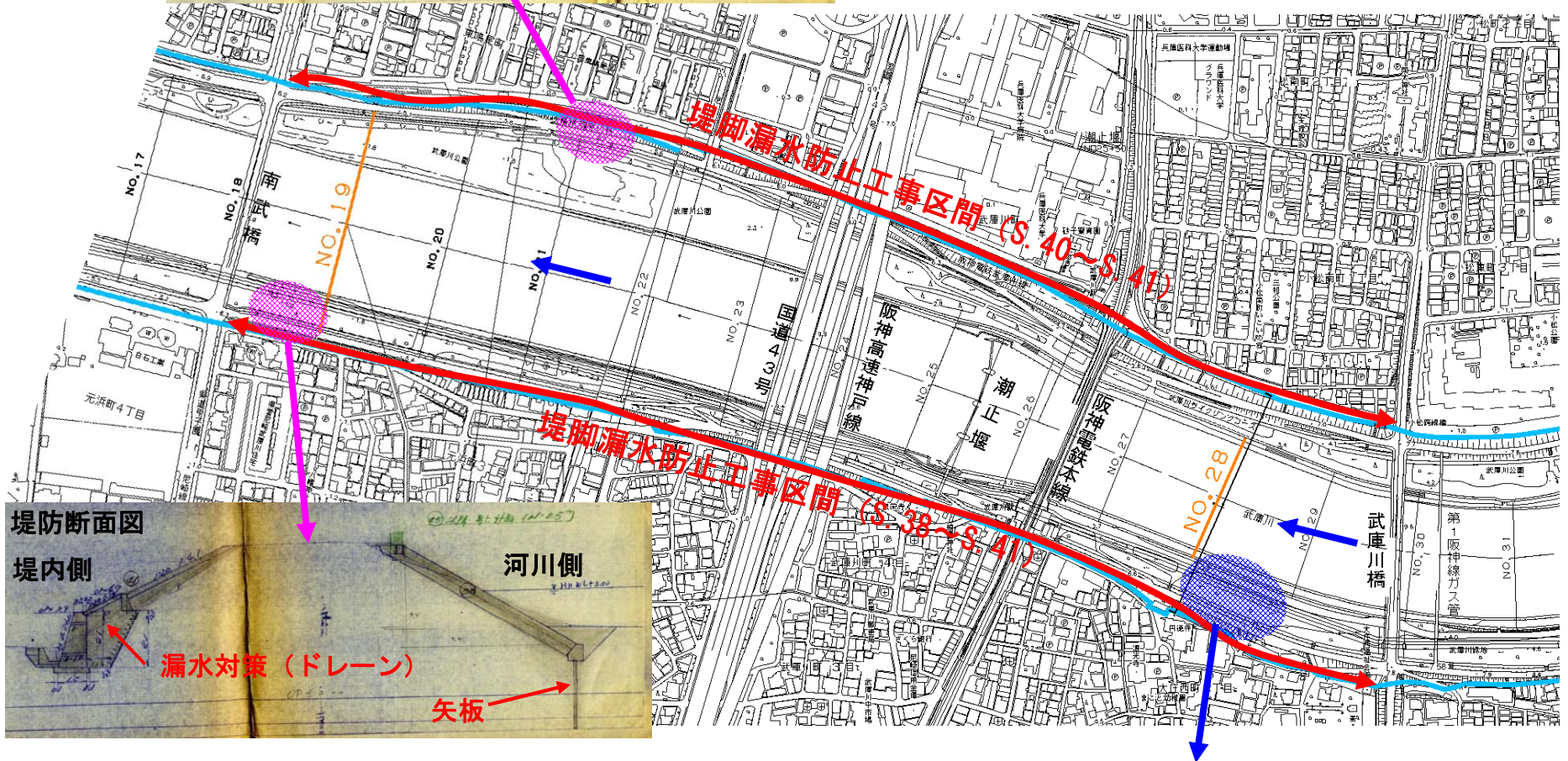
堤防強化工事の詳細調査の際、過去に施行した矢板及び漏水対策工が確認された箇所
