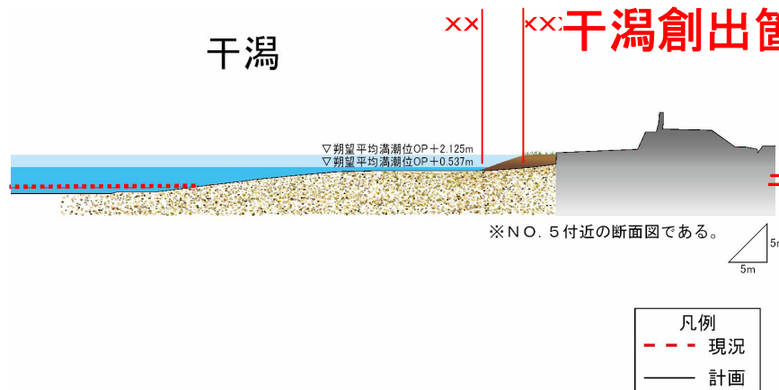
横断面図
