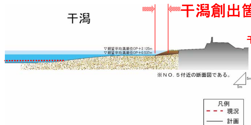
横断面図
