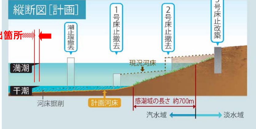
流下能力に余裕のある 箇所で干潟を創出
