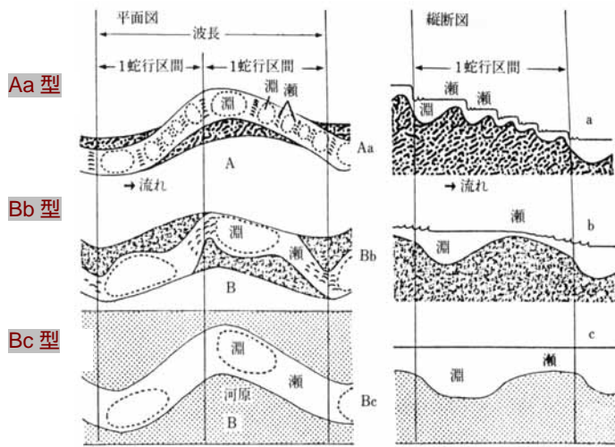
図 1.6.1 河川形態の基本的な3型の模式図
