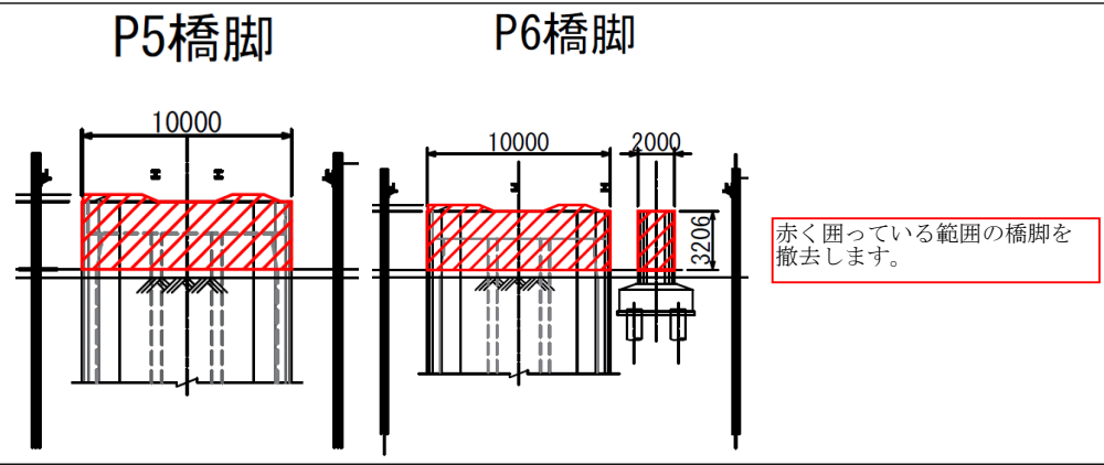
【断面図】
