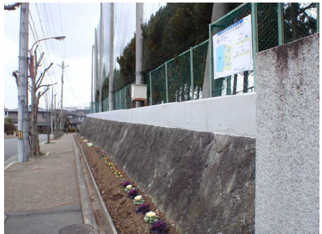
雨水貯留施設 (周囲小堤)
