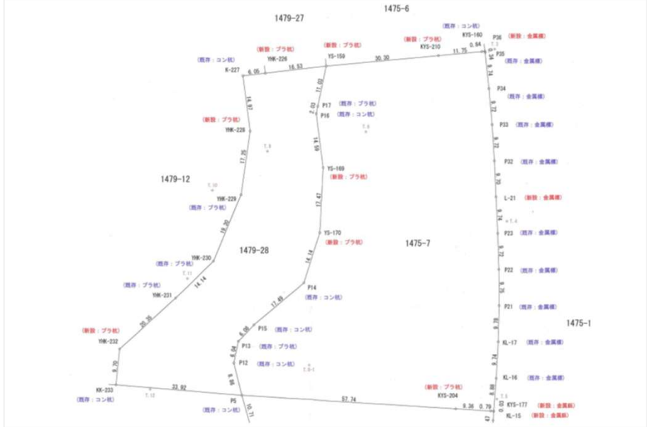
敷地形状図
