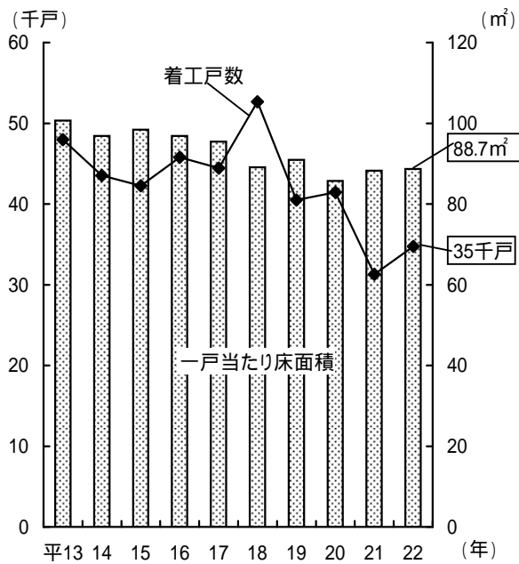
新設住宅着工戸数と平均床面積の推移
