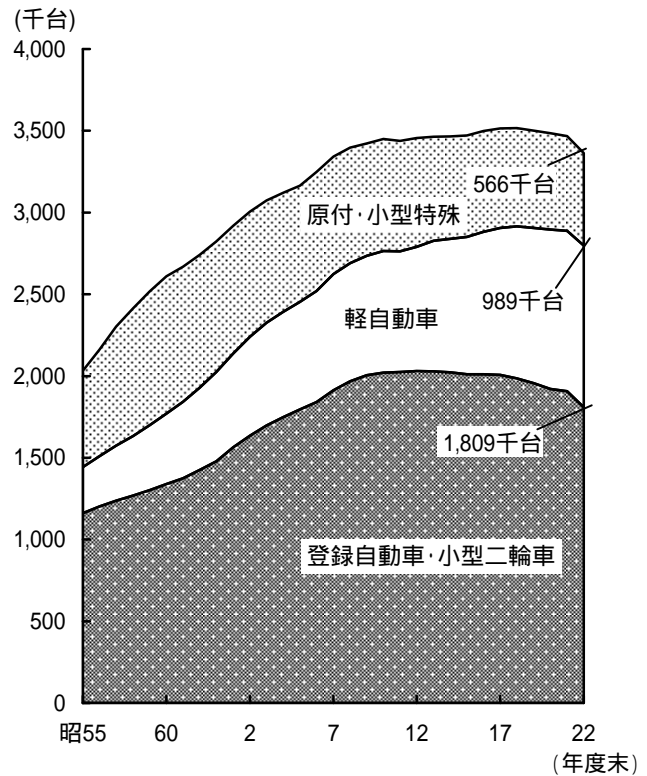
自動車台数の推移
