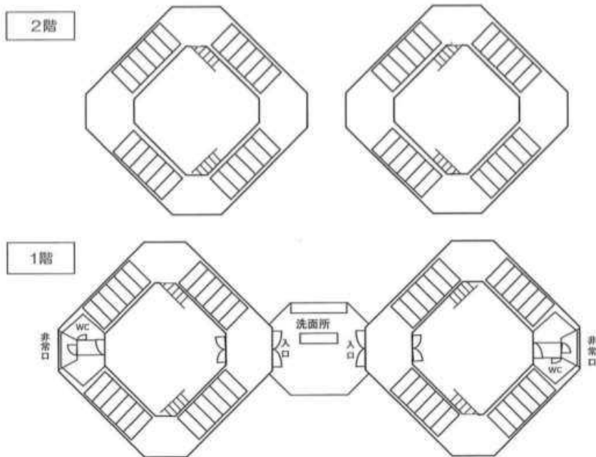
<青少年宿泊研修棟平面図>
