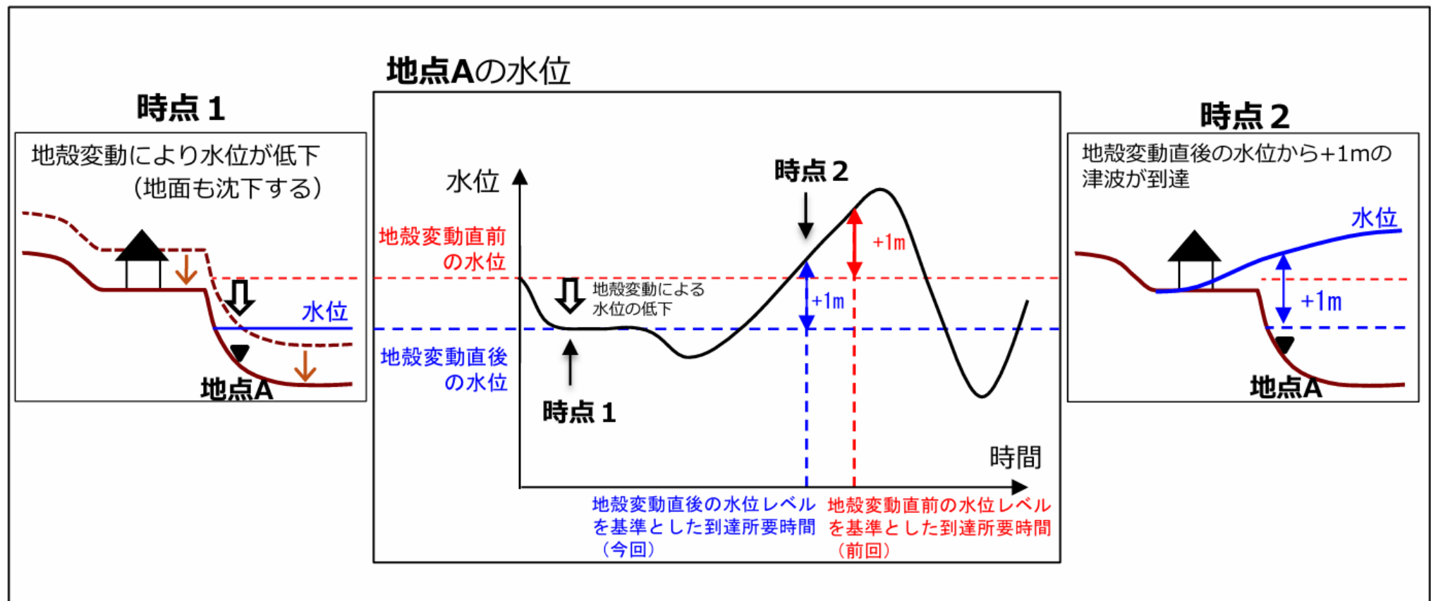
図3.12 沿岸における津波到達時間の計測方法の精査
