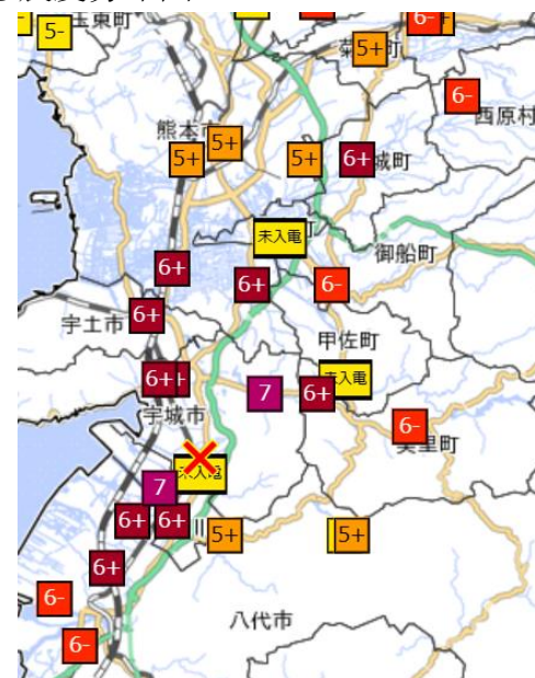
○震度分布図
