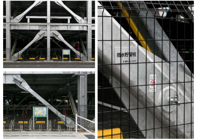
雨水貯留柱
