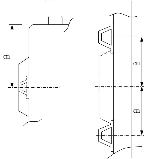
防舷材測定位置
