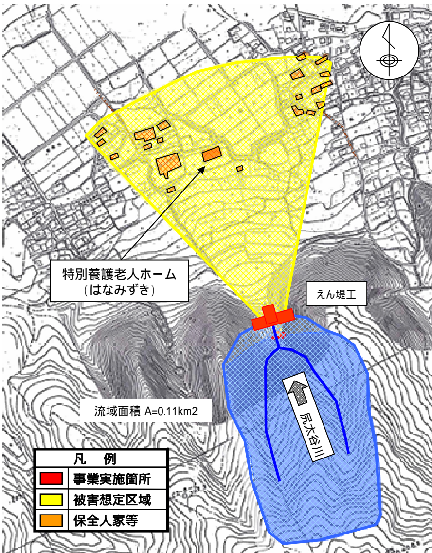
計画概略図 縮尺 1:10,000
