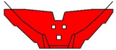
えん堤工 H=11.5m、L=70.0m
