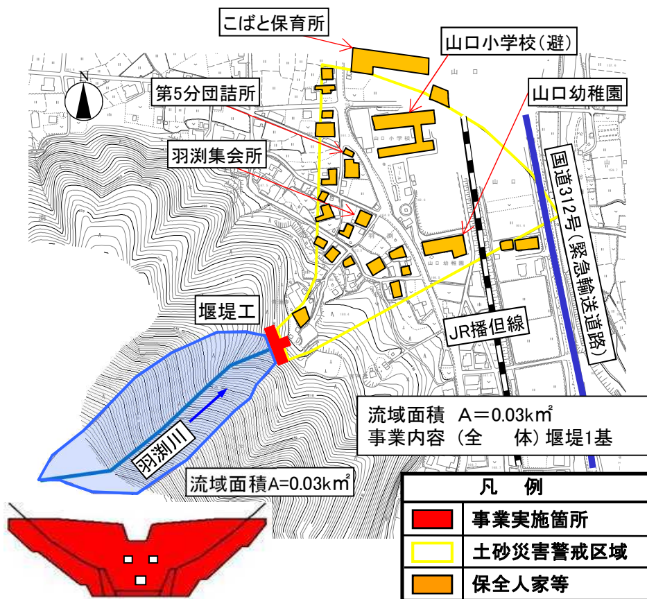
堰堤工 H=10.0m、L=50.0m
