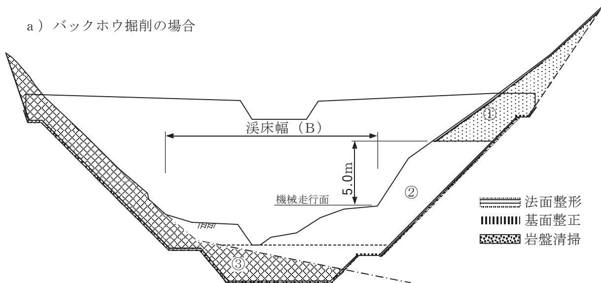
図－1 掘削区分
