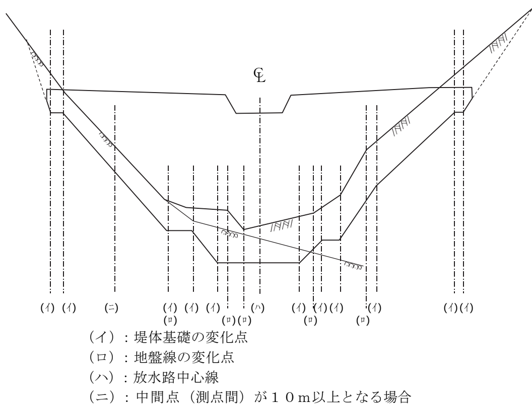
図一6 堤体軸直角方向の横断測点
