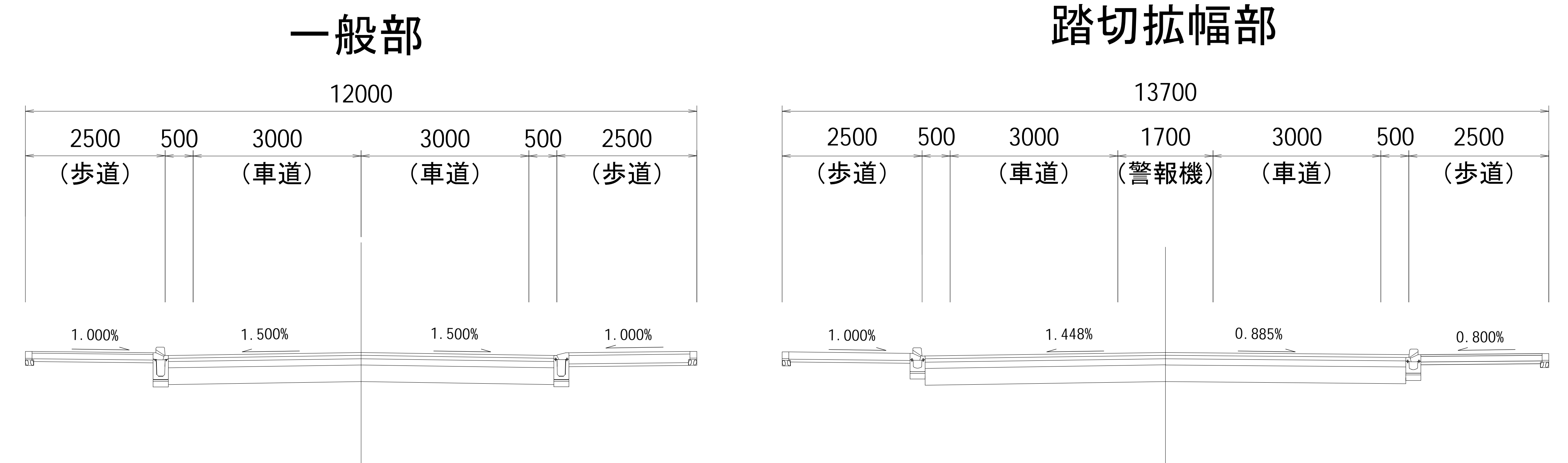
標準断面図
