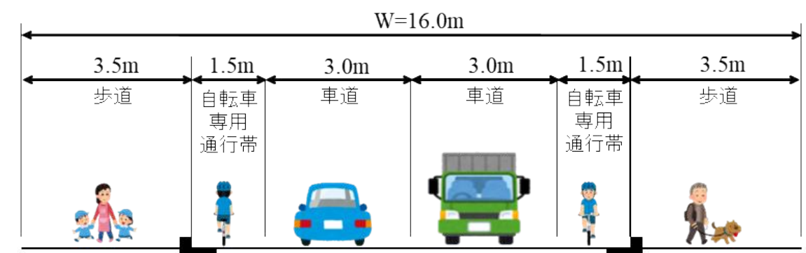
横断面図
