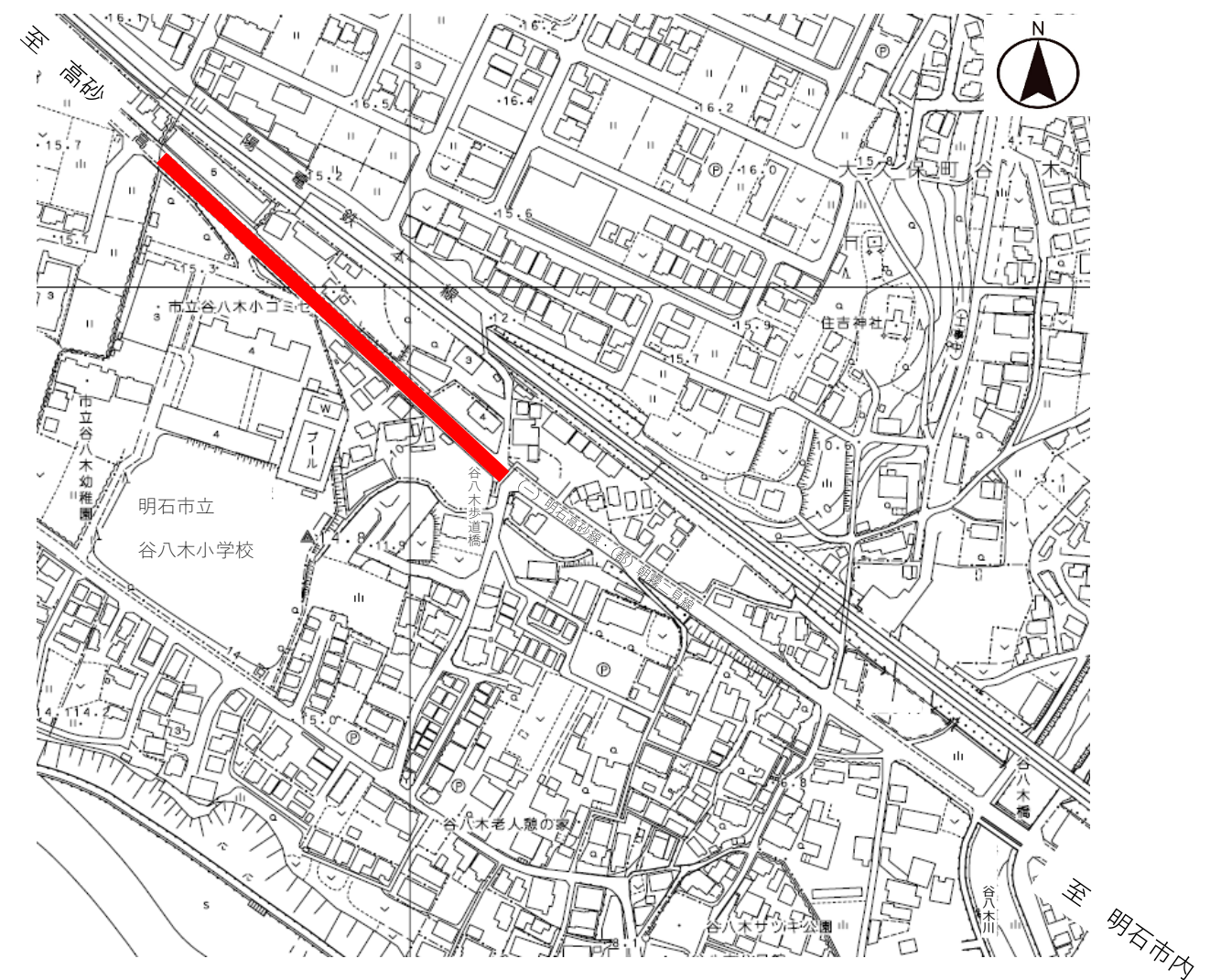
平面図
