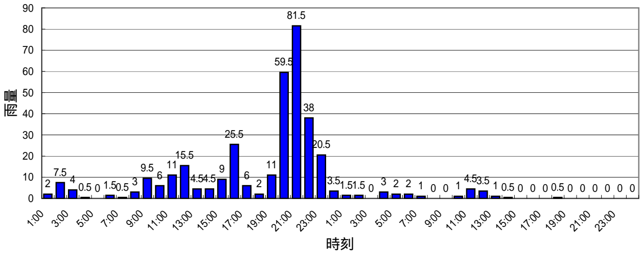
佐用(気象庁)地点 ハイエト
