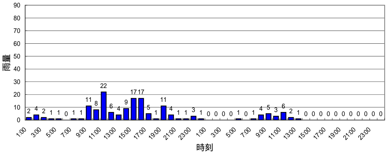
有年地点 ハイエト
