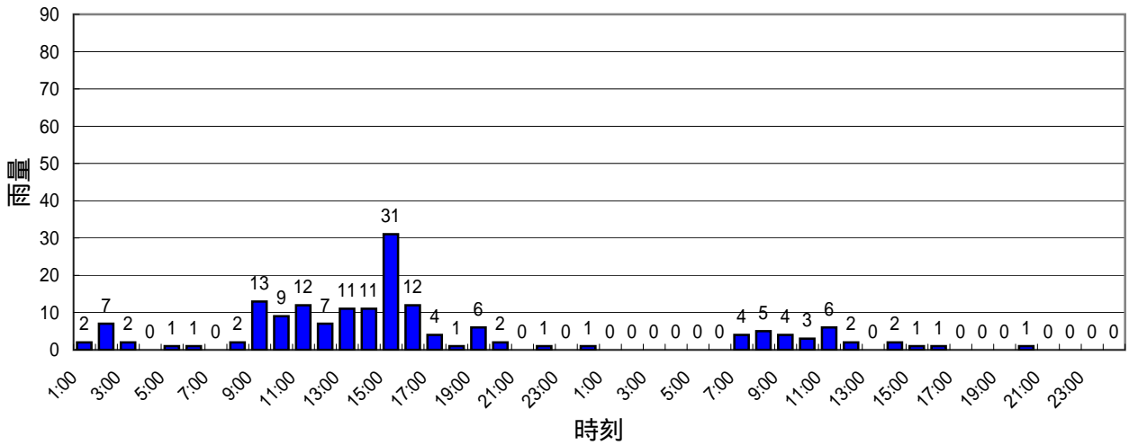
折方地点 ハイエト
