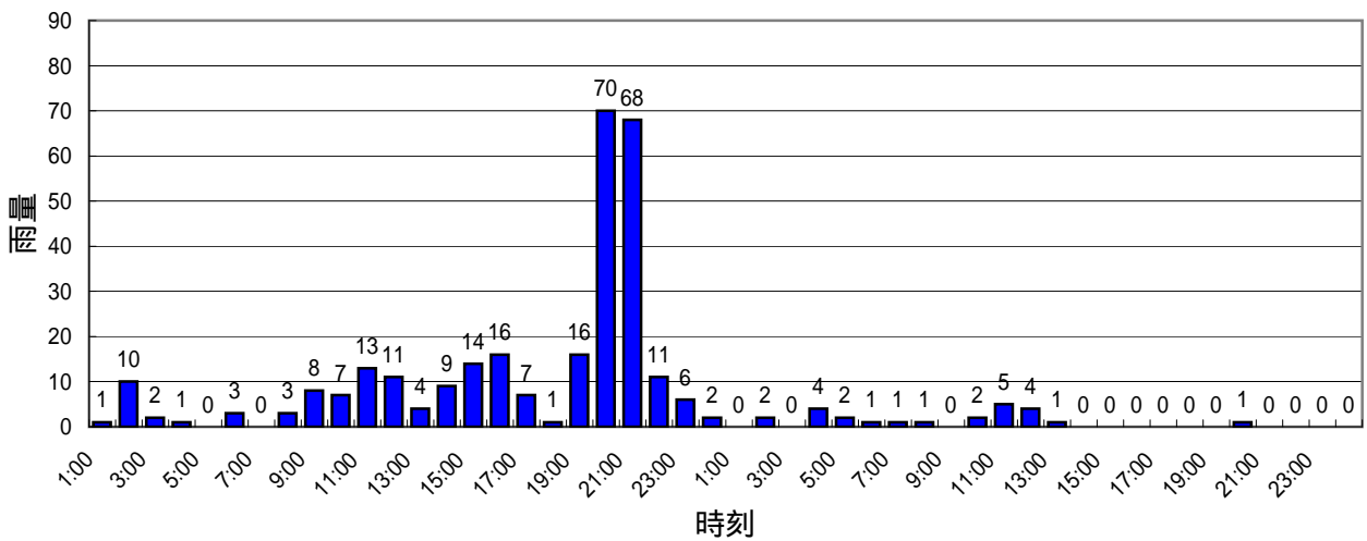
円光寺地点 ハイエト
