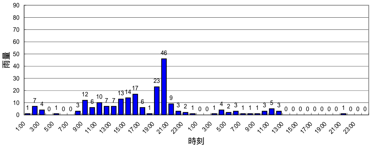
安室ダム地点 ハイエト
