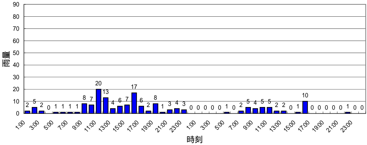
矢野地点 ハイエト
