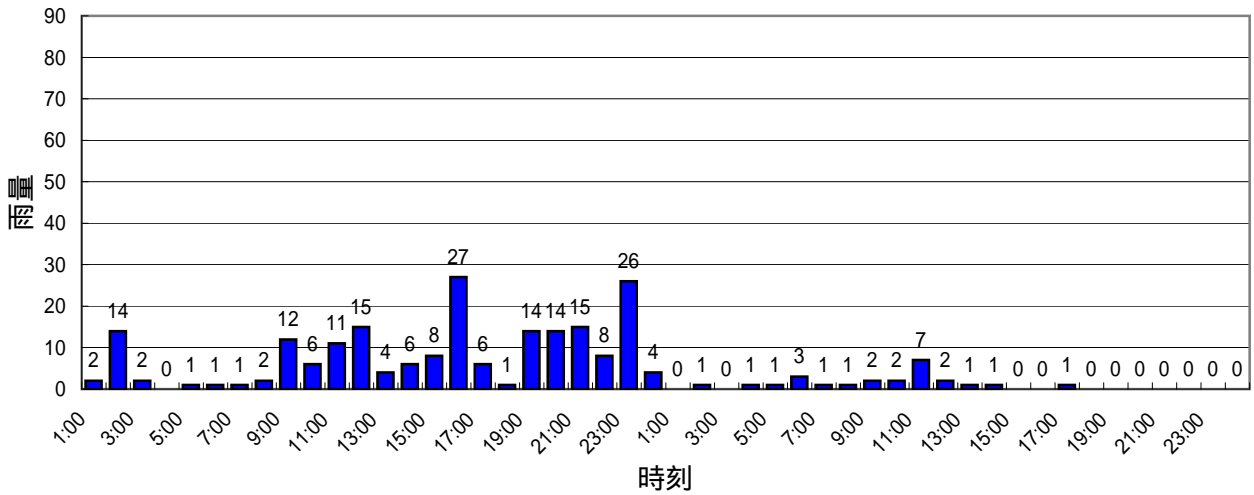
三日月地点 ハイエト
