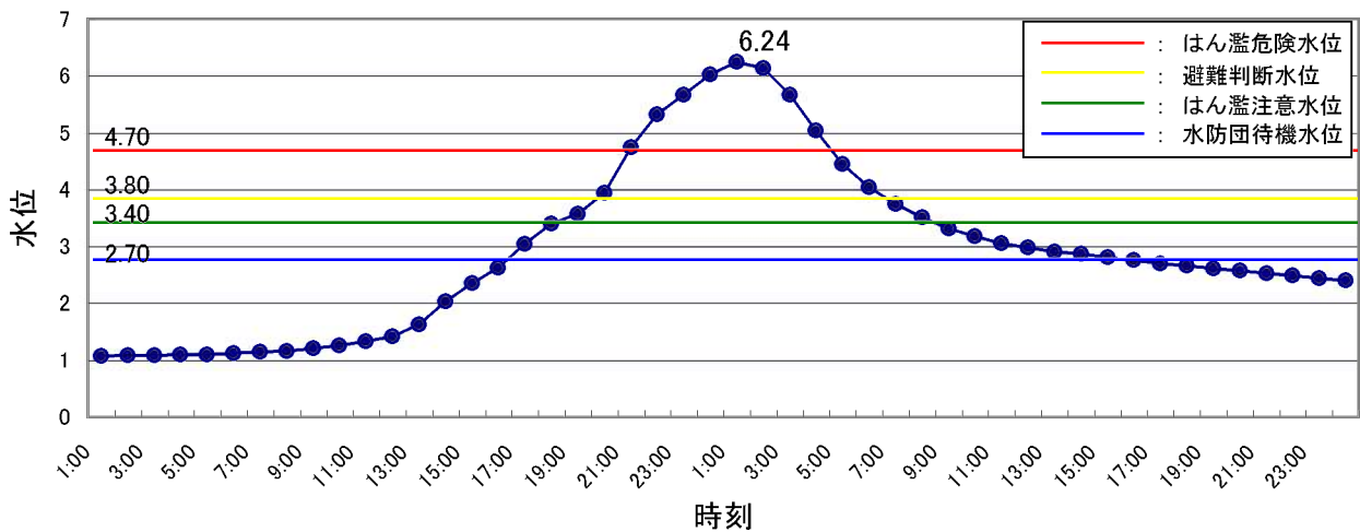
千種川(上郡) 水位ハイドロ
