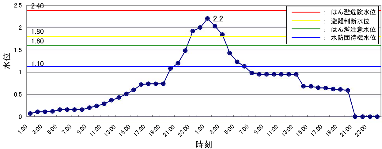
志文川(三日月) 水位ハイドロ
