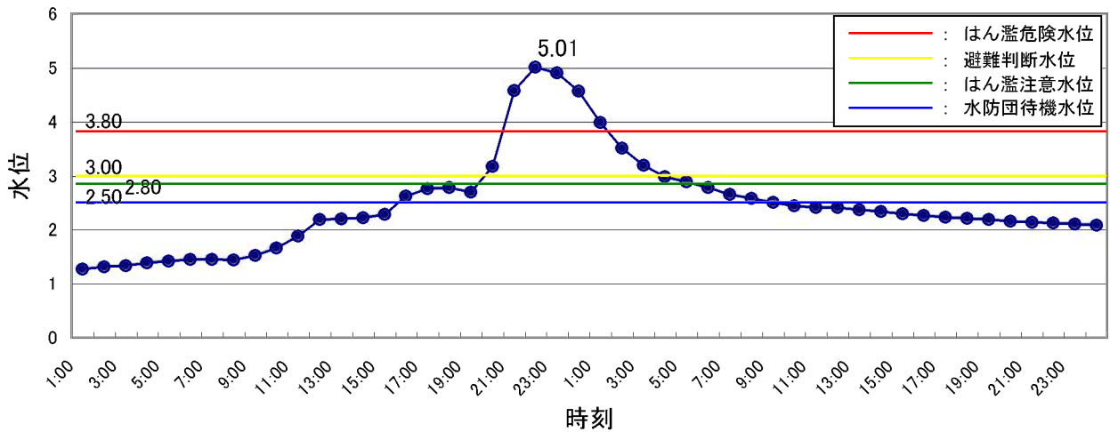
佐用川(佐用) 水位ハイドロ
