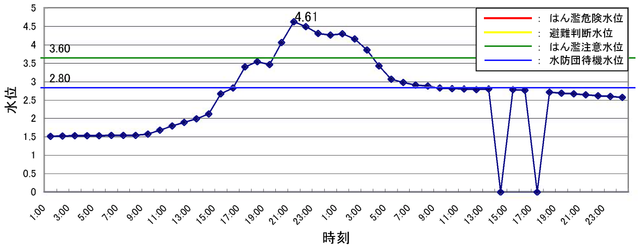
安室川(竹万) 水位ハイドロ
