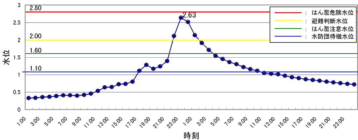
千種川(千種) 水位ハイドロ
