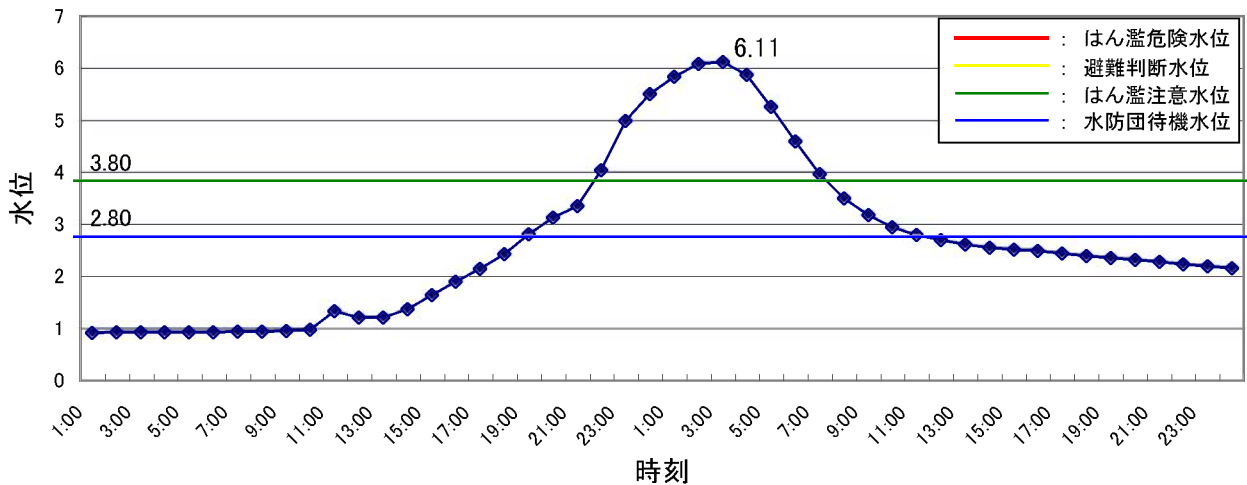
千種川(木津) 水位ハイドロ
