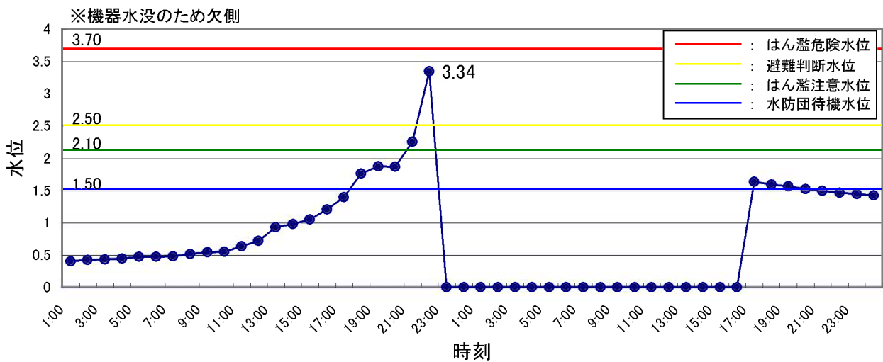
千種川(上三河) 水位ハイドロ
