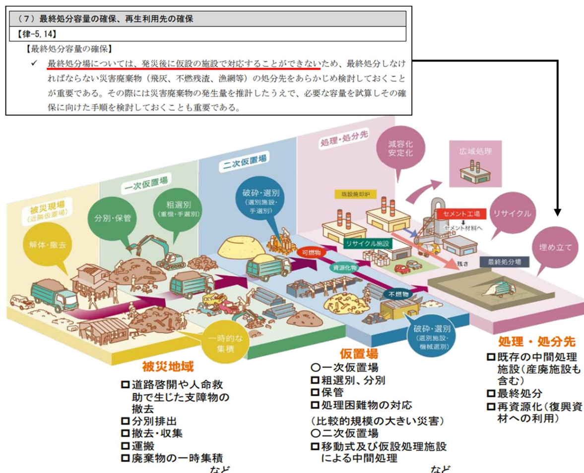
図 2.4.37 災害廃棄物の処理フロー
