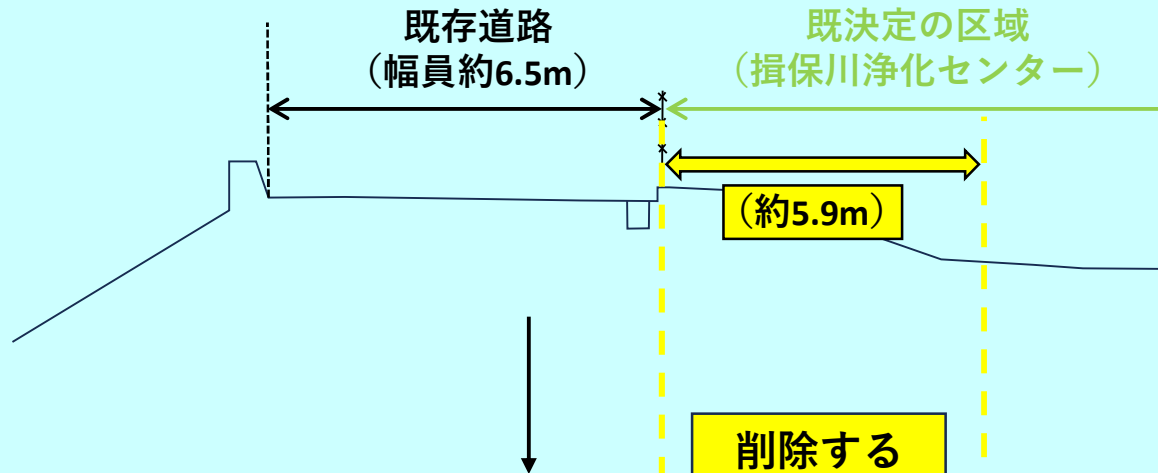
現況横断図
