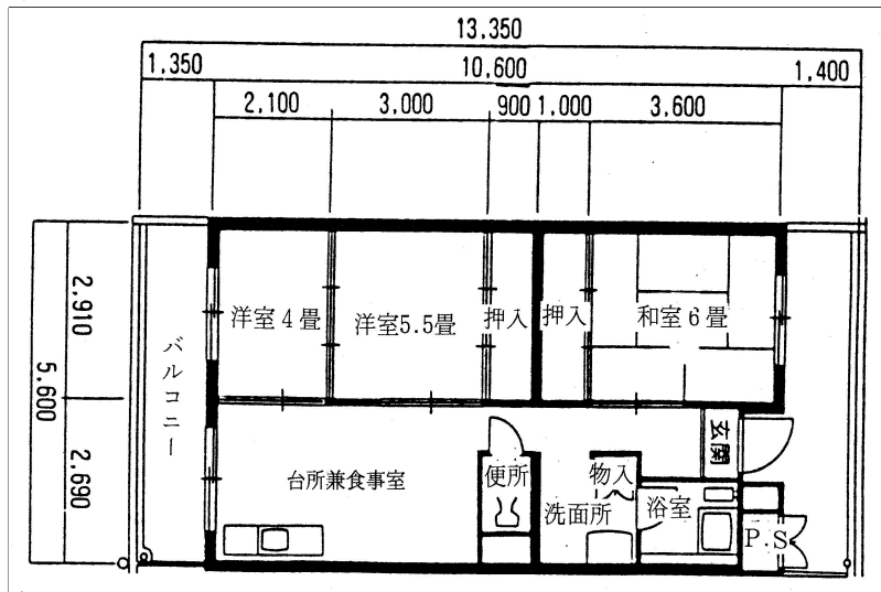
住戸図
