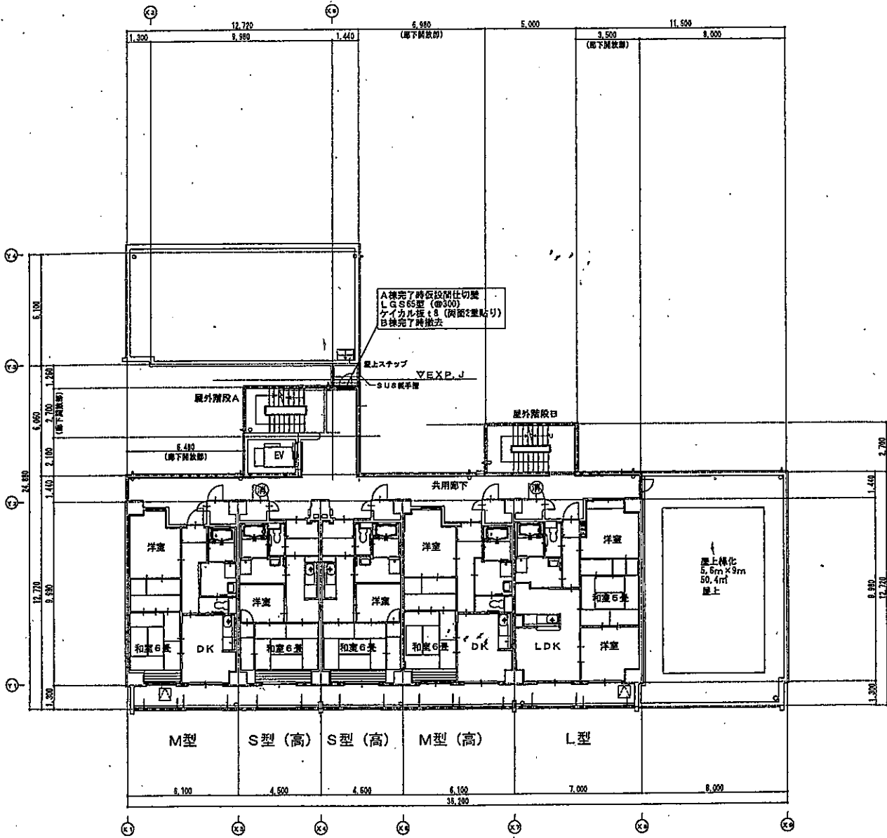
7階平面図 1/200
