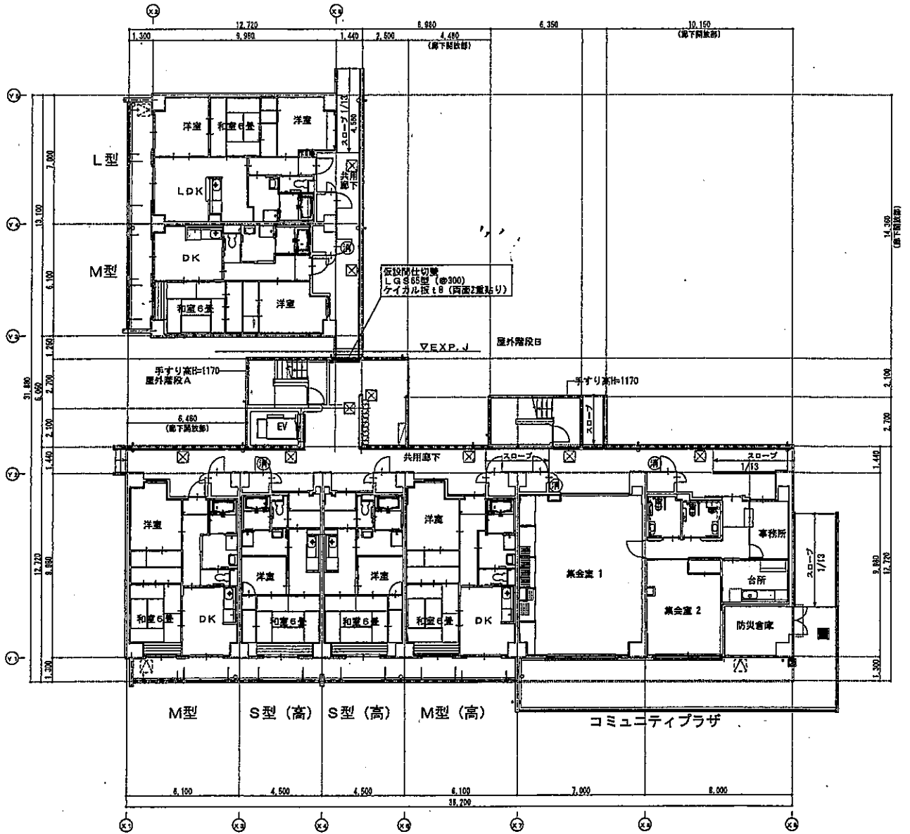
1階平面図 1/200
