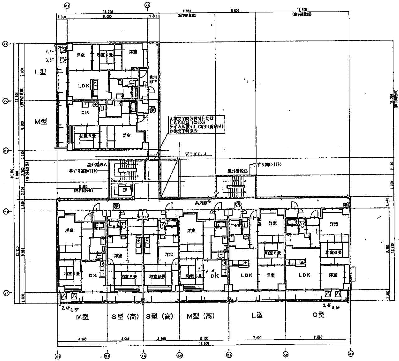
2階~5階平面図 1/200
