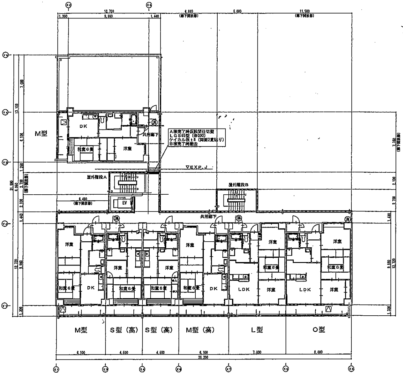
6階平面図 1/200
