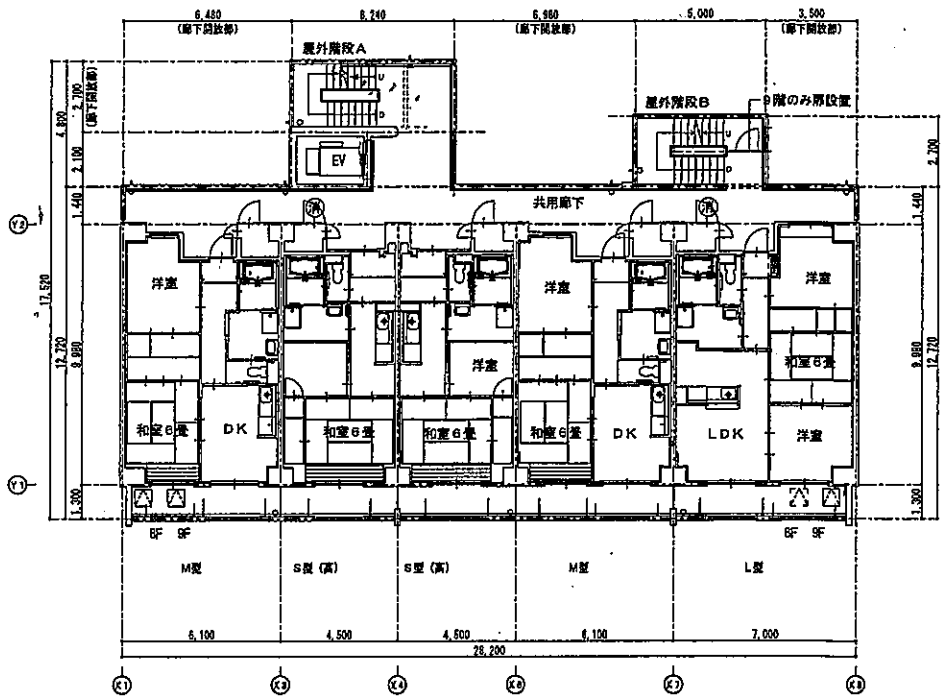
8階~9階平面図 1/200
