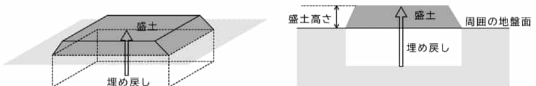
図1-1-3 窪地における盛土の取扱い
