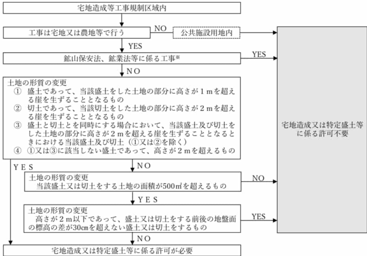
※ 「2 許可を要しない宅地造成等に関する工事」参照 図3-2-1 宅地造成等工事規制区域における宅地造成又は特定盛土等に関する工事の許可の要否判断フロー
