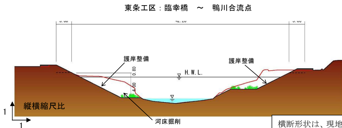
図 2.1.32 東条川整備横断イメージ (1)
