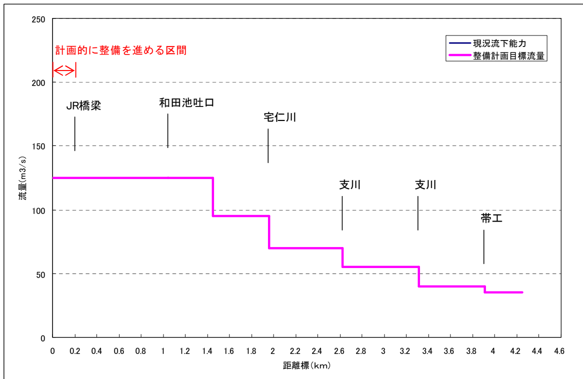
図 2. 1. 42 油谷川流下能力縦断面図
