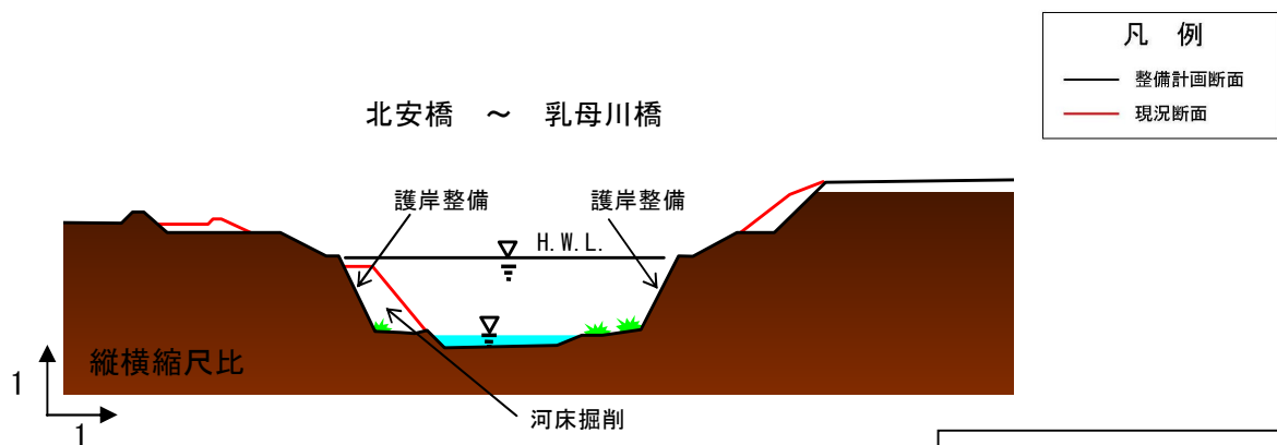
図 2.1.60 奥荒田川整備横断イメージ
