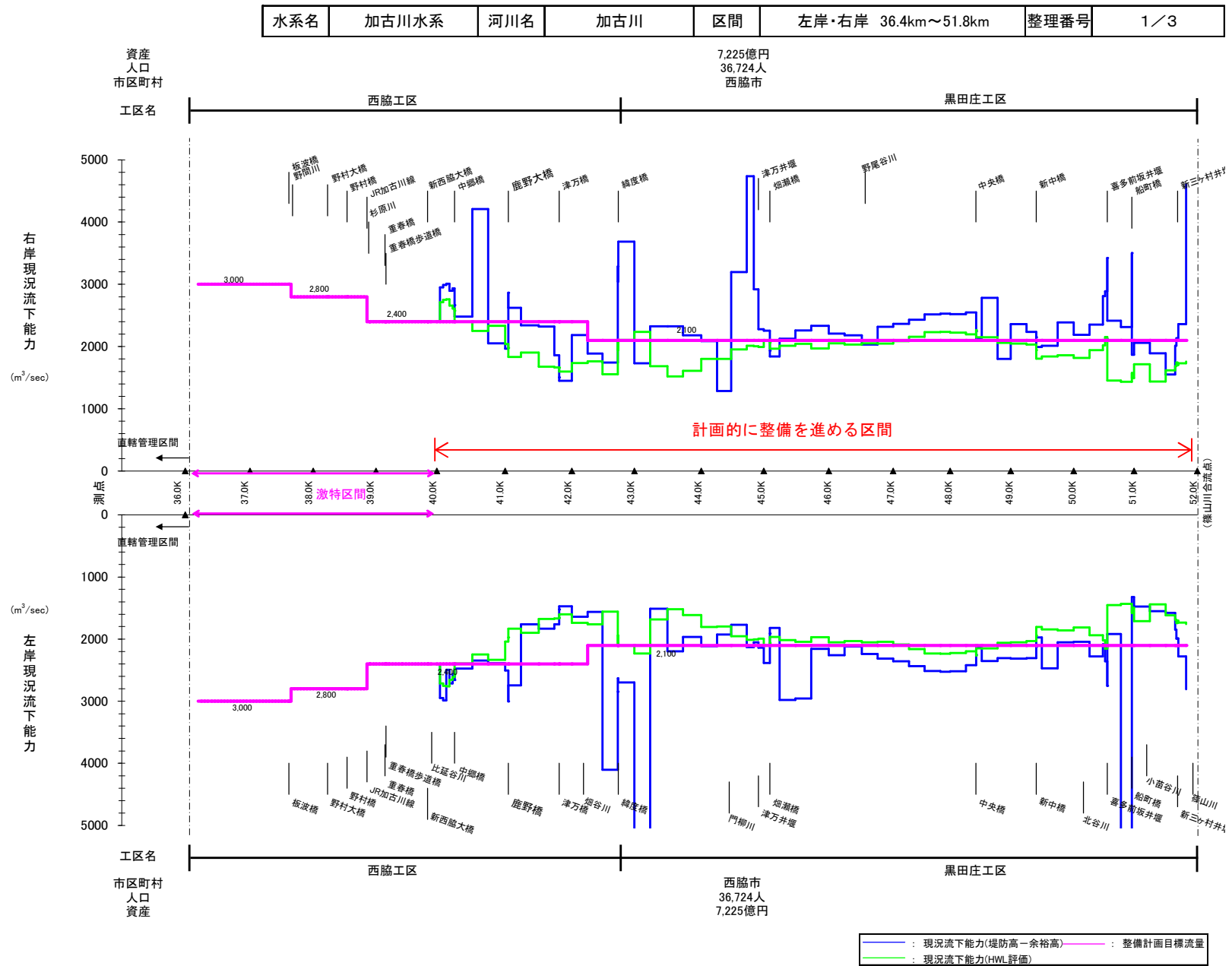
図 2.1.2 加古川流下能力縦断図
