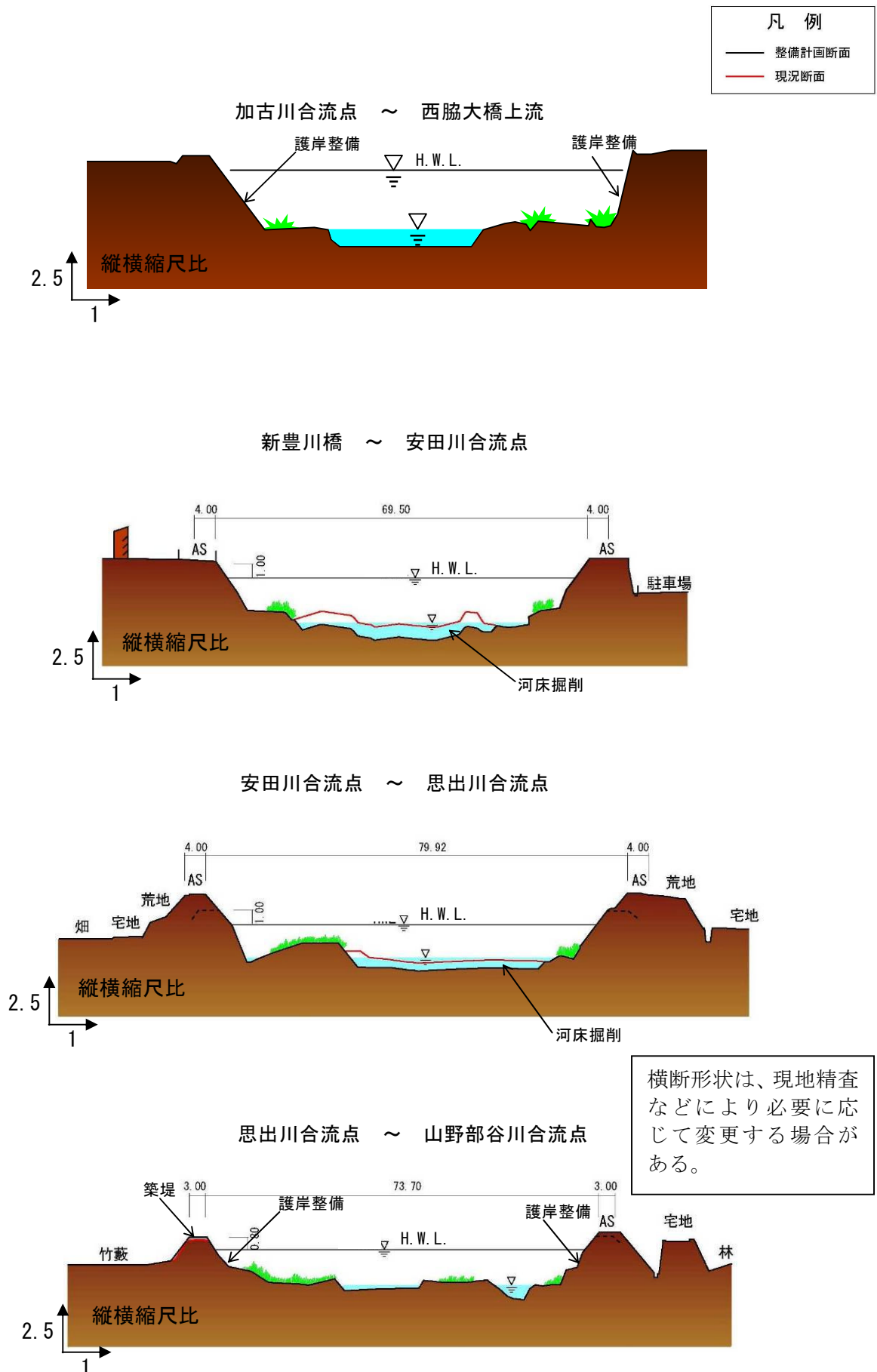
図 2.1.52 杉原川整備横断イメージ (1)
