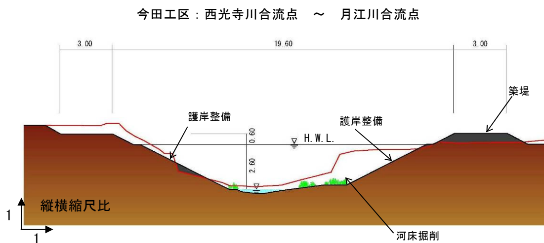
図 2.1.32 東条川整備横断イメージ (2)
