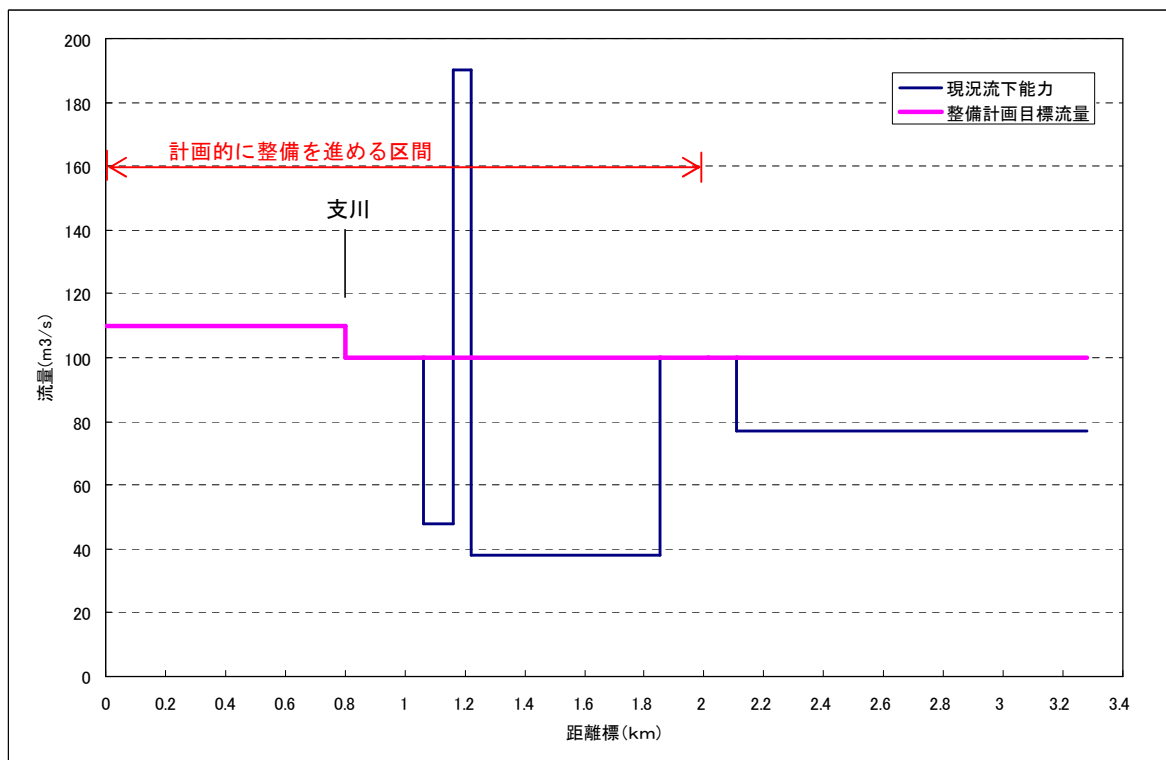
図 2. 1. 54 思出川流下能力縦断図
