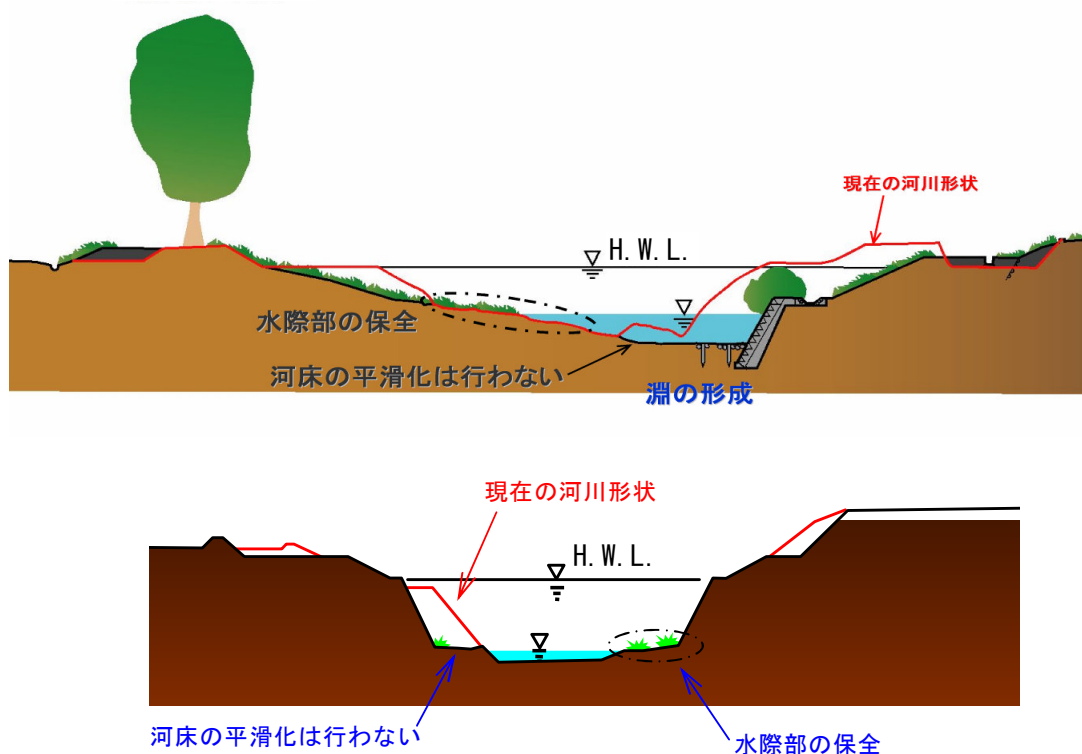
図 2.1.61 河道改修後のイメージ
