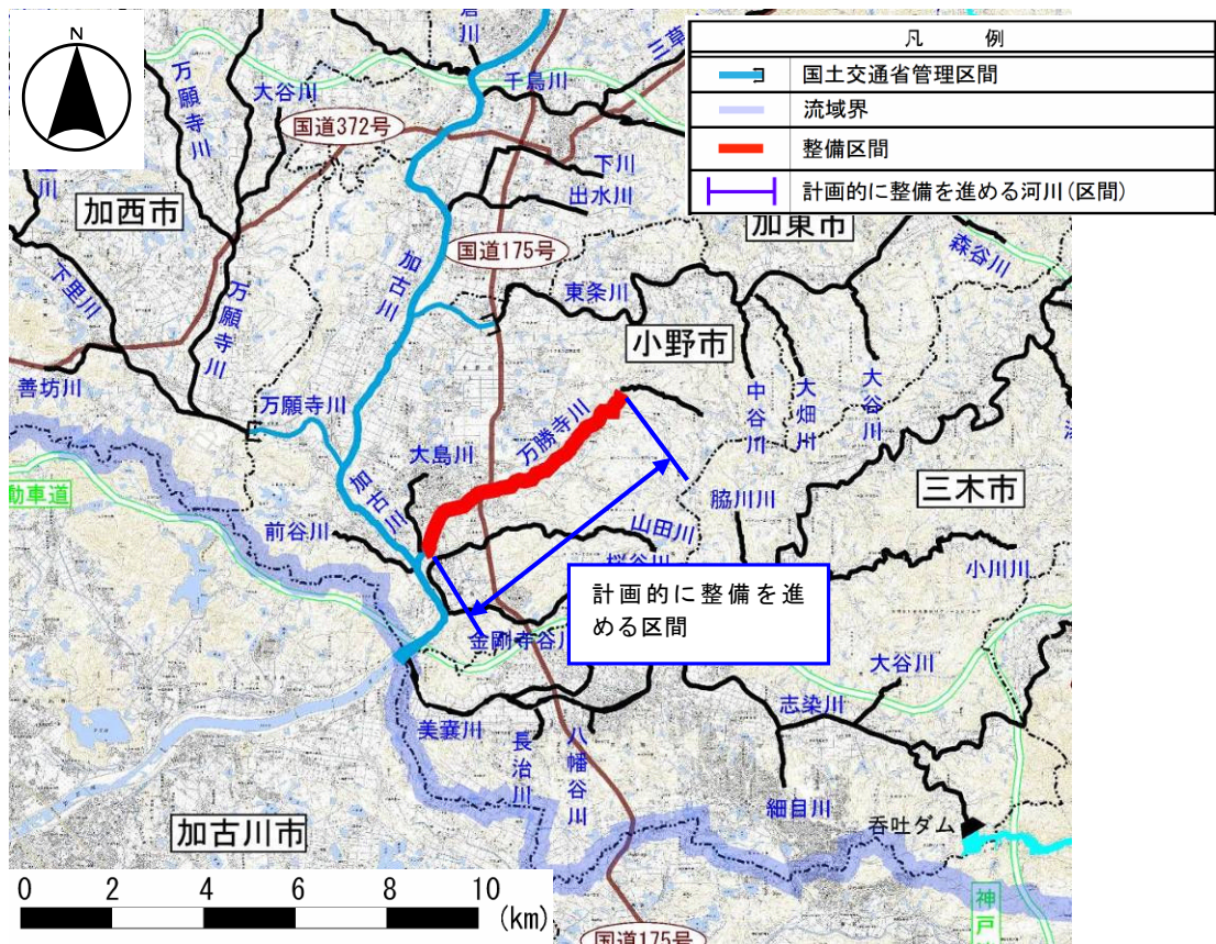
図 2.1.25 河川整備計画対象区間（万勝寺川）
