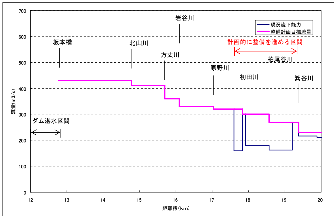
図 2.1.10 志染川流下能力縦断面図
