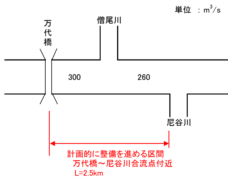
図 2.1.15 淡河川整備計画目標流量配分
