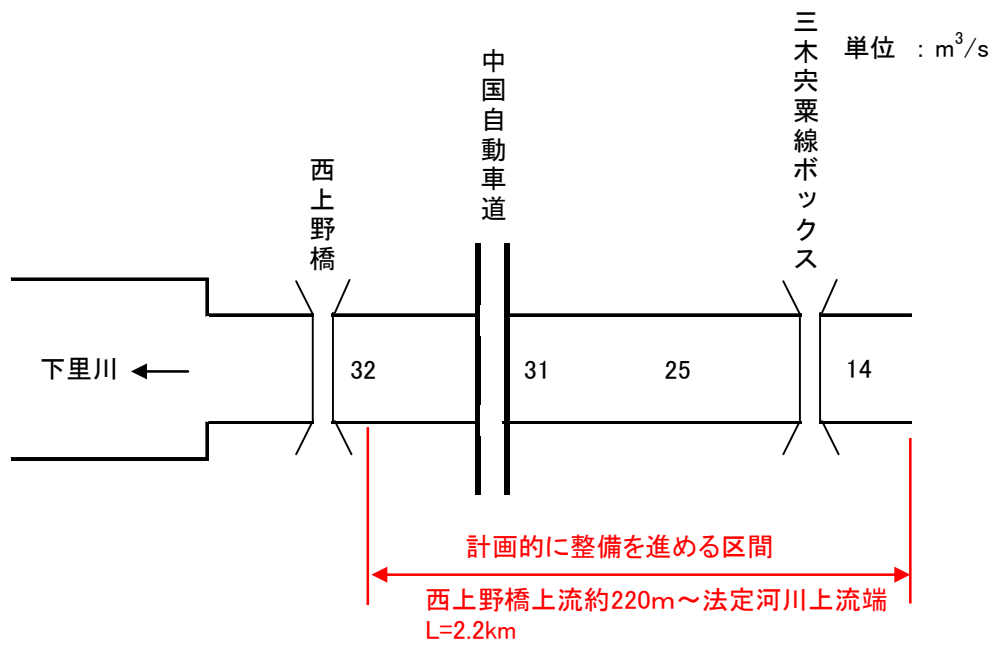
図 2.1.19 千歳川整備計画目標流量配分
