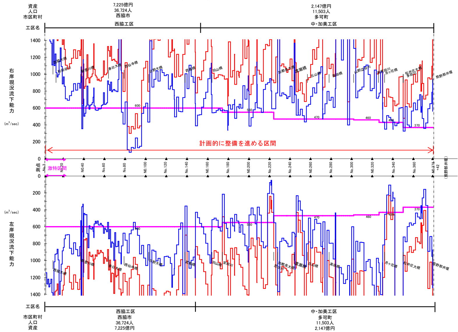
図 2.1.50 杉原川流下能力縦断面図
