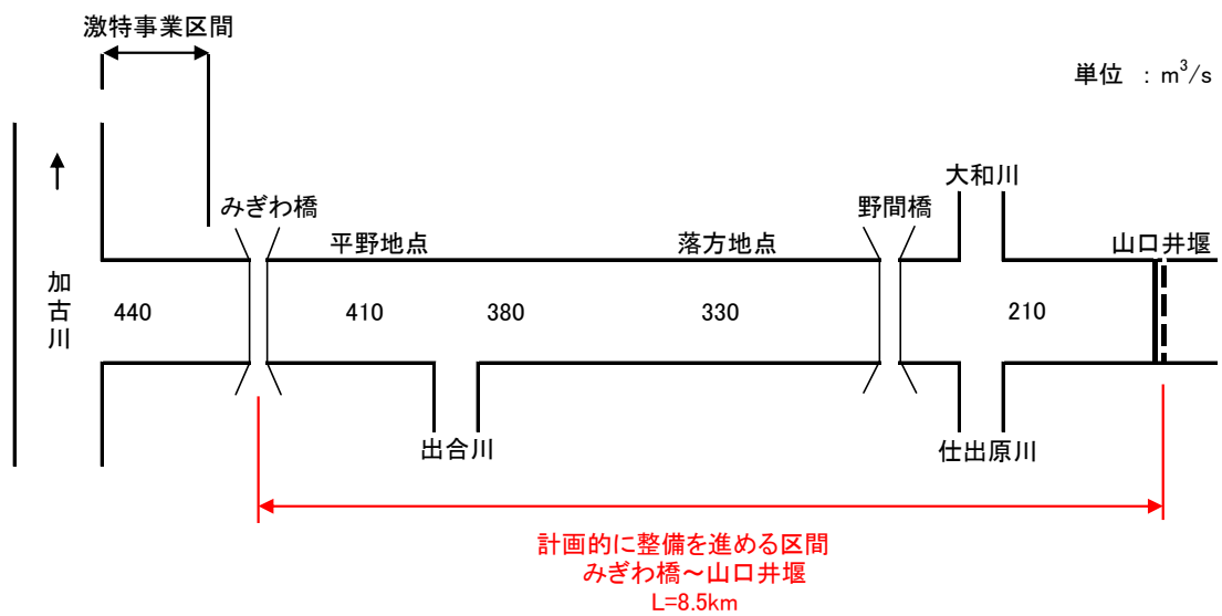
図 2.1.47 野間川整備計画目標流量配分
