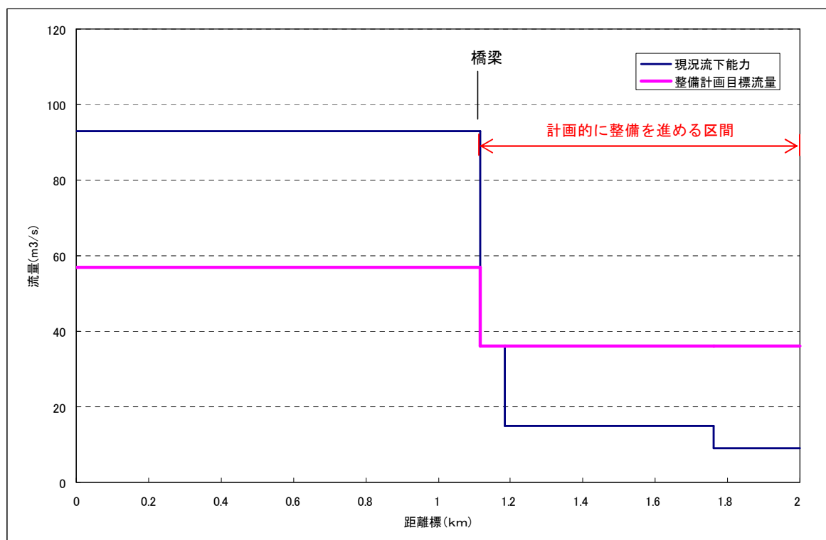
図 2.1.34 大谷川流下能力縦断面図
