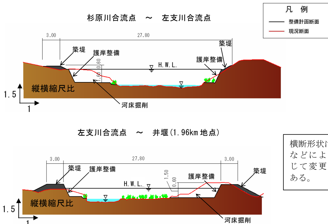
図 2.1.56 思出川整備横断イメージ
