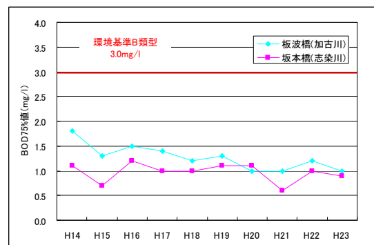
図 1.2.2 河川水質(BOD)の経年変化
