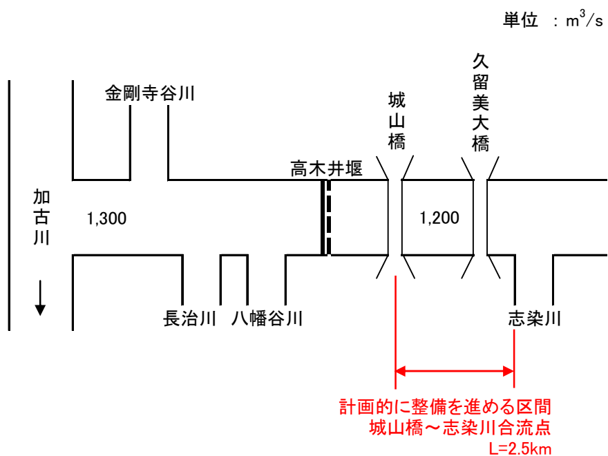
図 2.1.7 美囊川整備計画目標流量配分
