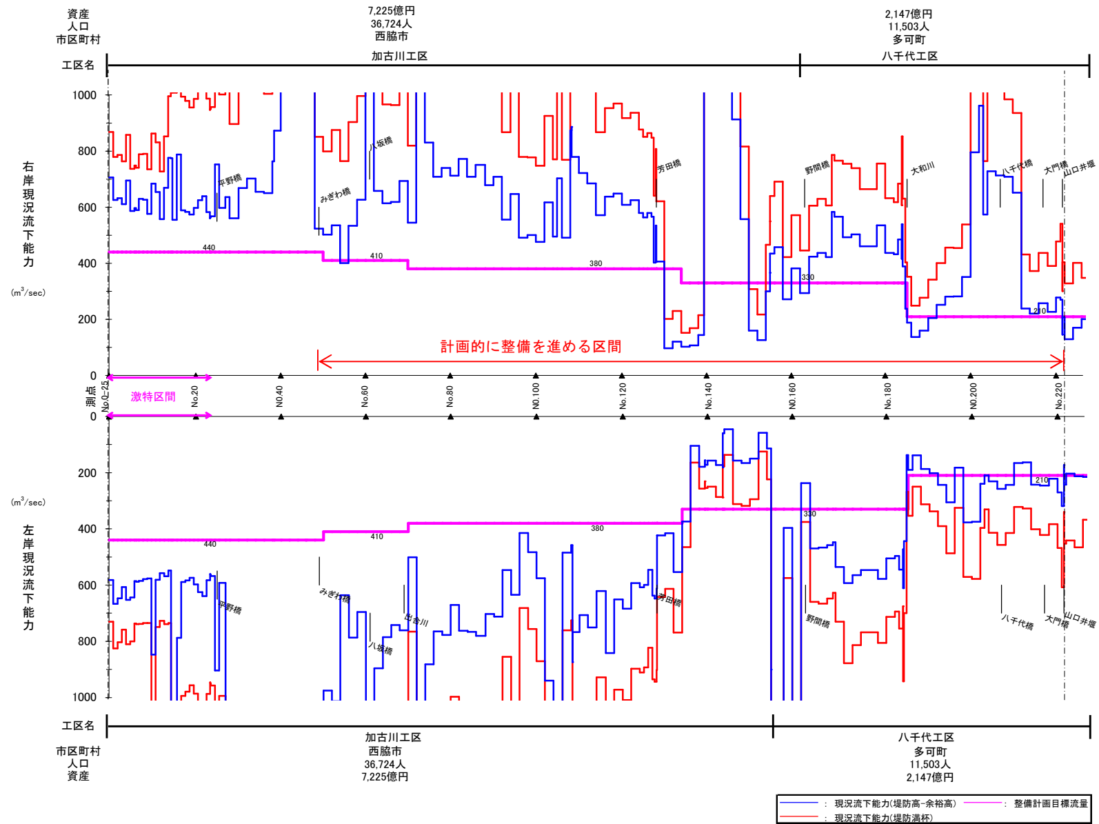
図 2.1.46 野間川流下能力縦断面図
