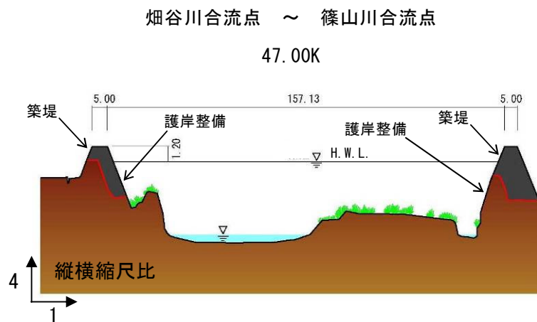
図 2.1.4 加古川整備横断イメージ
