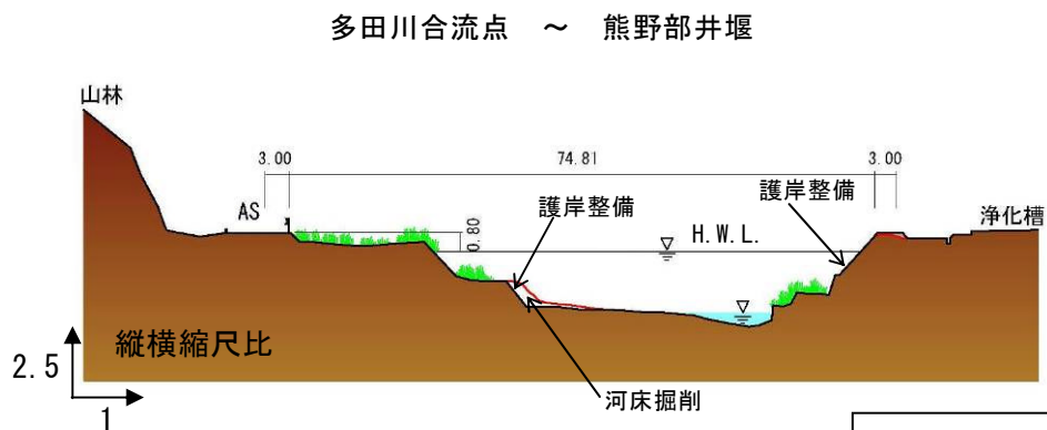
図 2.1.52 杉原川整備横断イメージ (2)
