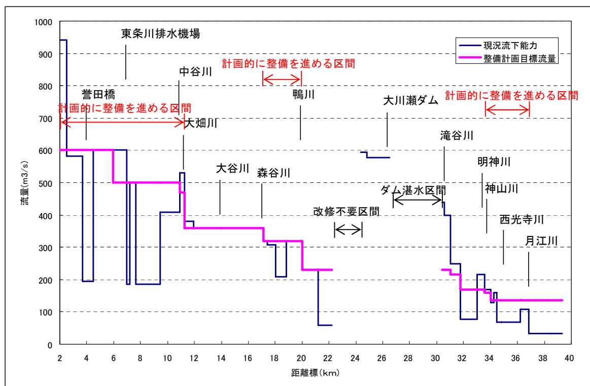
図 2. 1. 30 東条川流下能力縦断図
