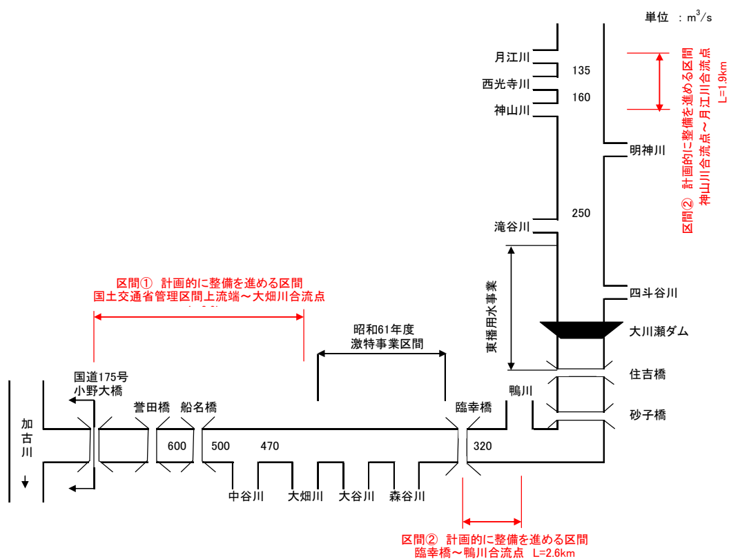
図 2. 1. 31 東条川整備計画流量配分
