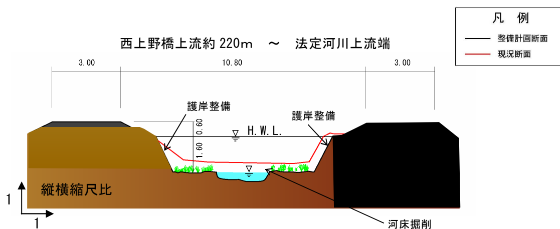
図 2.1.20 千歳川整備横断イメージ
