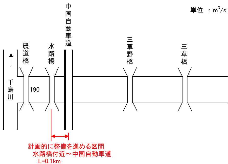
図 2.1.39 三草川整備計画目標流量配分
