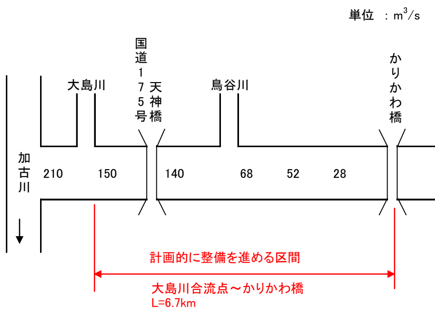
図 2.1.27 万勝寺川整備計画目標流量配分
