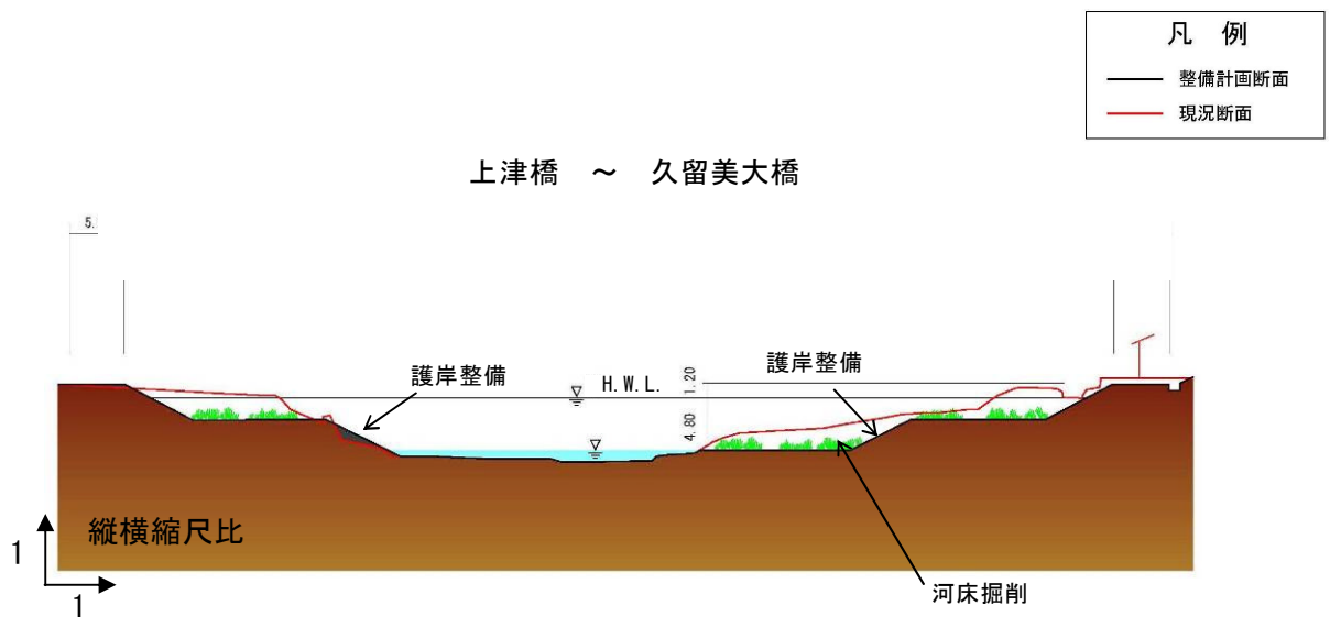
図 2.1.8 美囊川整備横断イメージ
