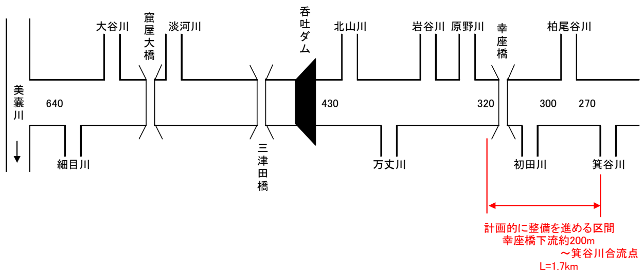
図 2.1.11 志染川整備計画目標流量配分
