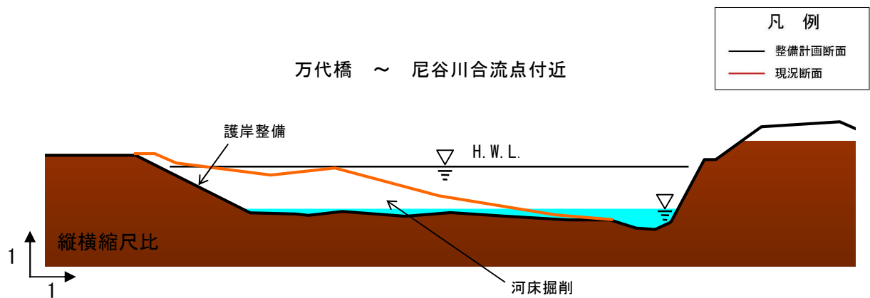
図 2.1.16 淡河川整備横断イメージ
