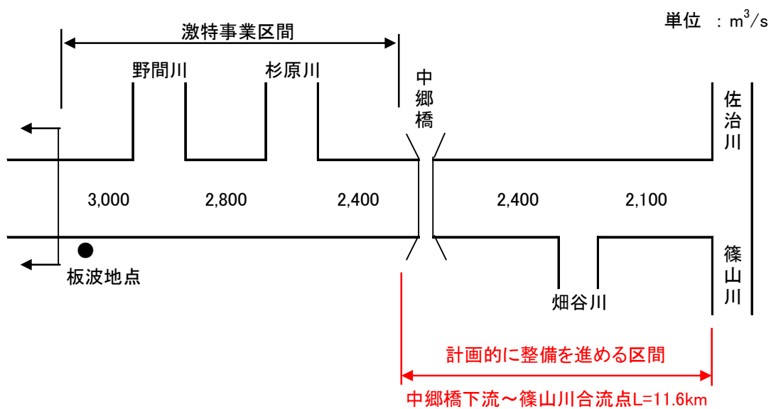
図 2. 1. 3 加古川整備計画目標流量配分
