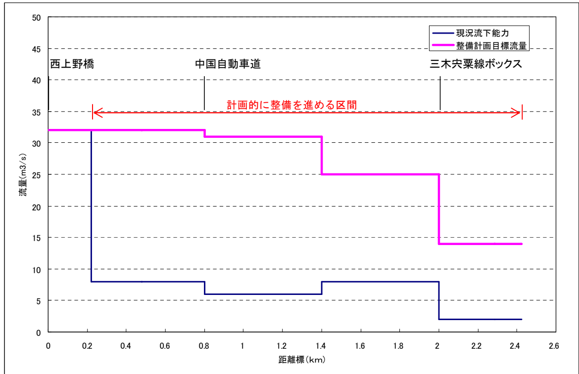
図 2.1.18 千歳川流下能力縦断図
