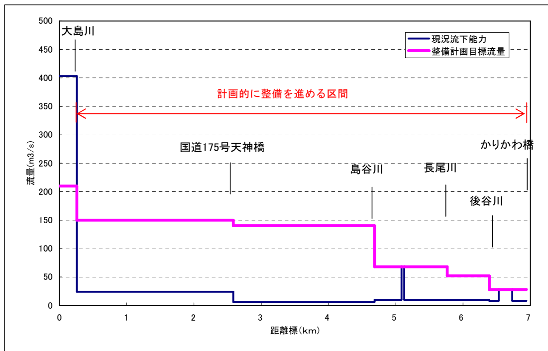
図 2.1.26 万勝寺川流下能力縦断面図
