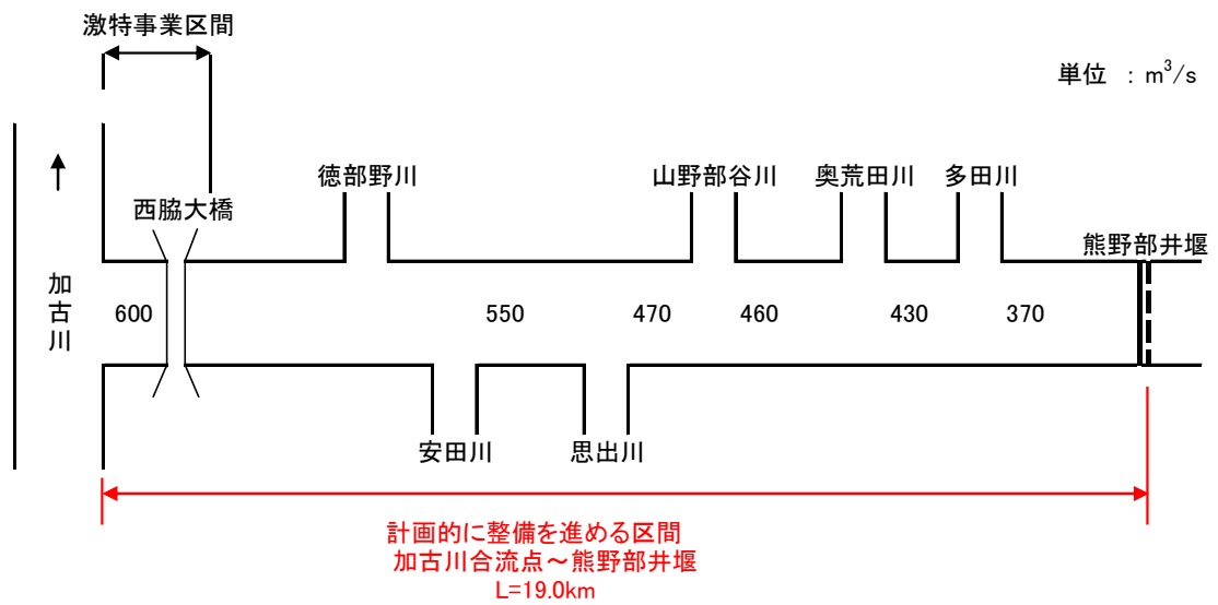
図 2. 1. 51 杉原川整備計画目標流量配分
