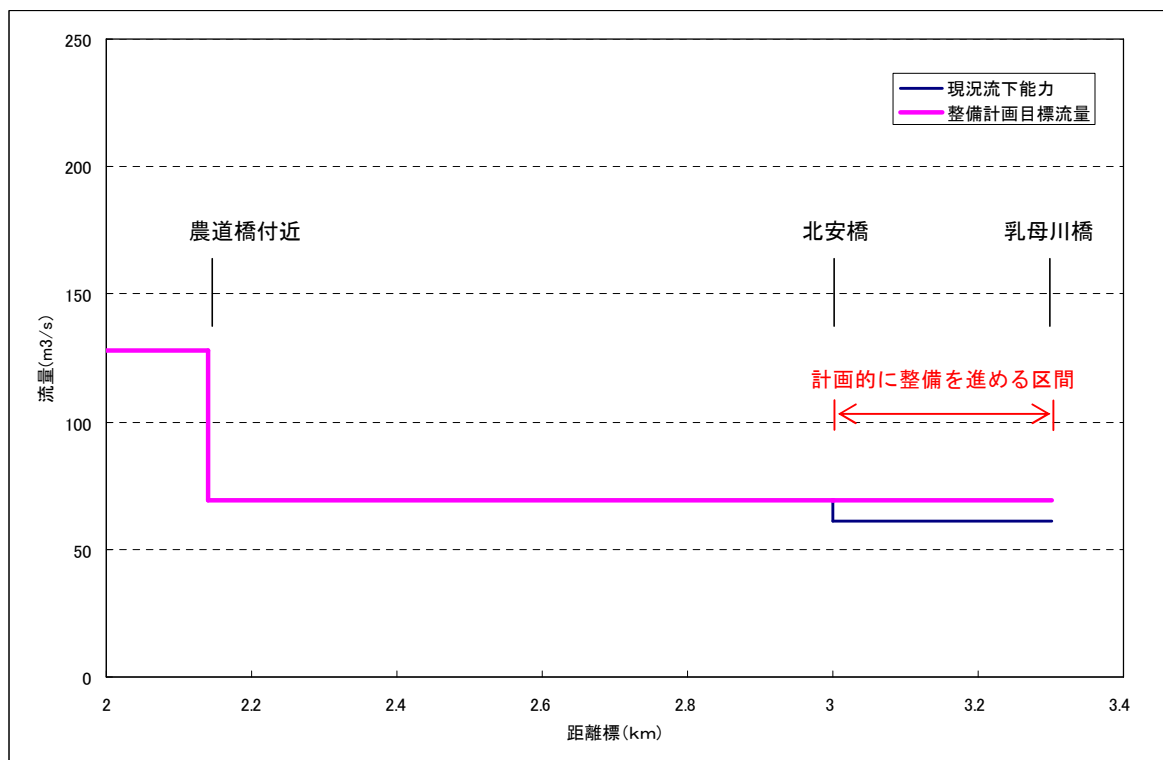
図 2.1.58 奥荒田川流下能力縦断図
