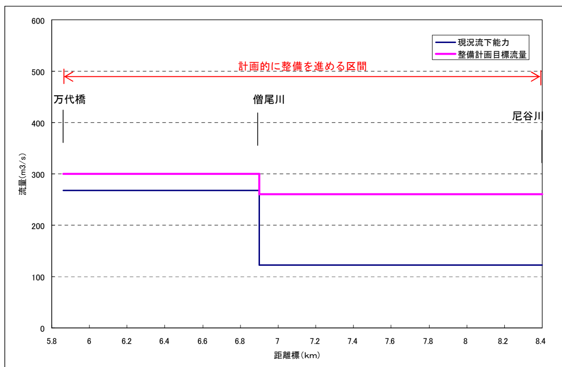
図 2.1.14 淡河川流下能力縦断面図
