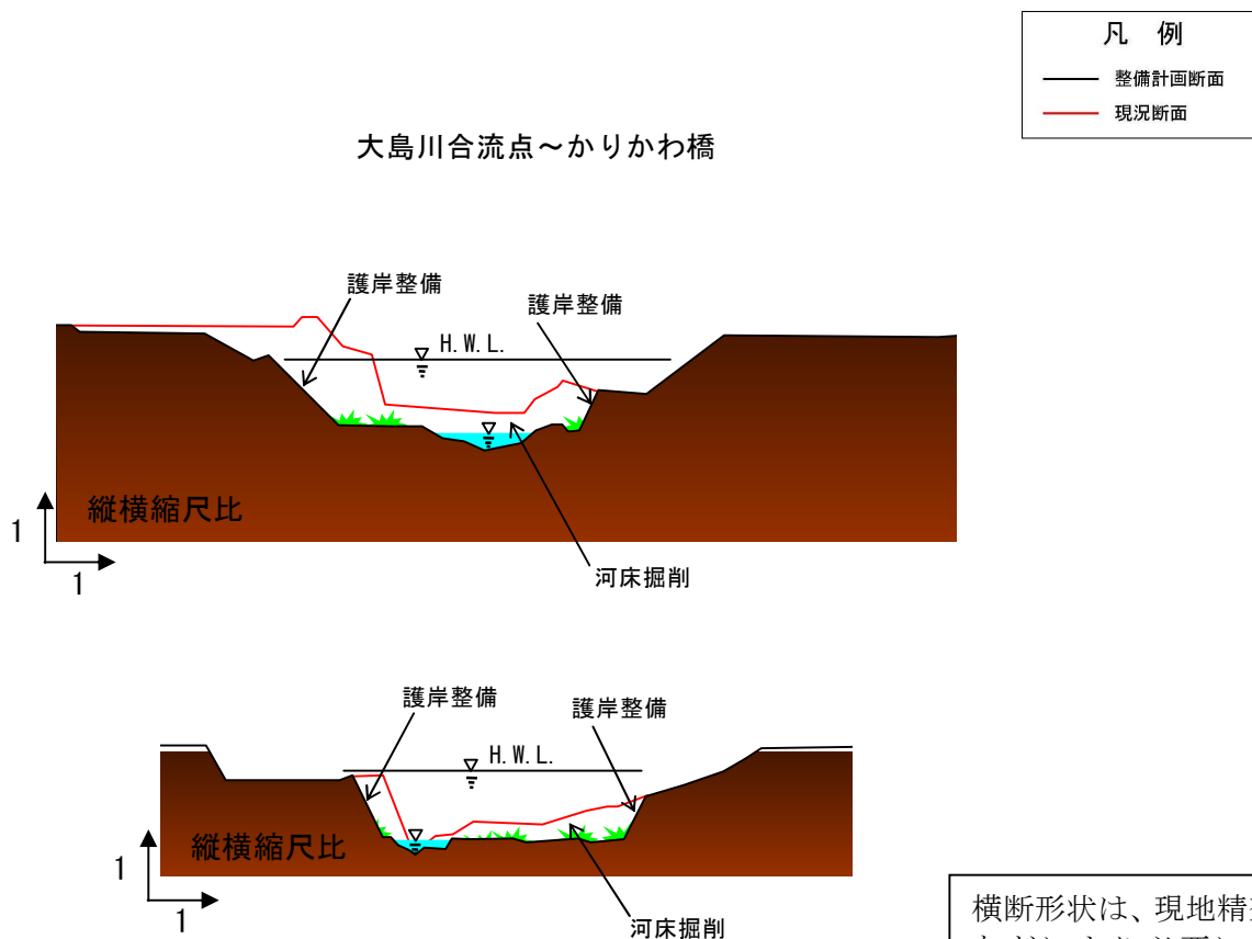
図 2.1.28 万勝寺川整備横断イメージ
