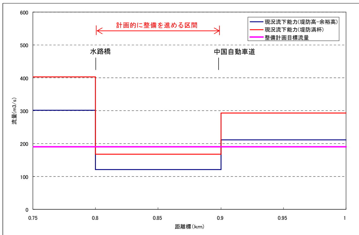
図 2.1.38 三草川流下能力縦断図
