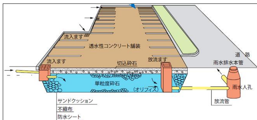
図 45 公園貯留浸透施設
