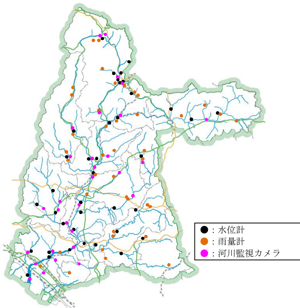
図 58 水位・雨量計・河川監視カメラ位置図
