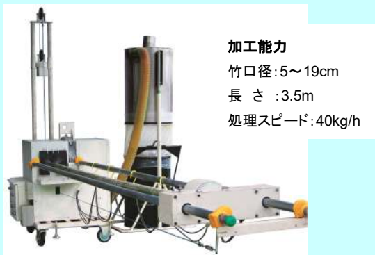
竹粉碎機「バンブーミル」
