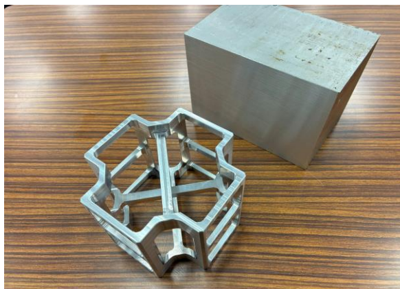
【5軸マシニングセンタ加工例】
