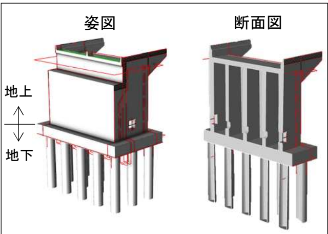
(参考) 橋台完成時のイメージ
