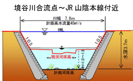
図 1.3.9 香住谷川の改修計画断面の例
