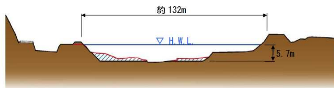
図 1.3.11 矢田川の改修計画断面の例
