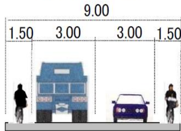
【計画横断面図】
